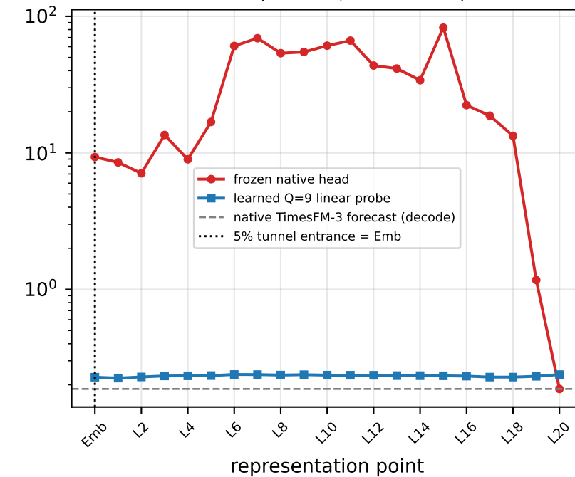
BOOM (PT-OOD, test N=354)
