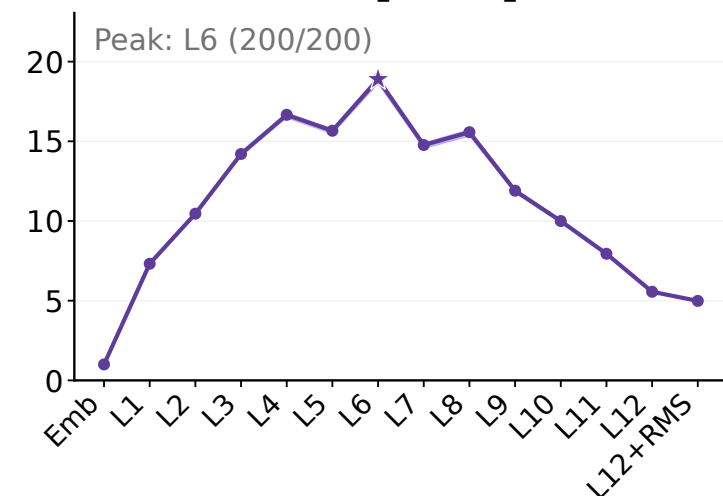
M4 [PT-ID]
