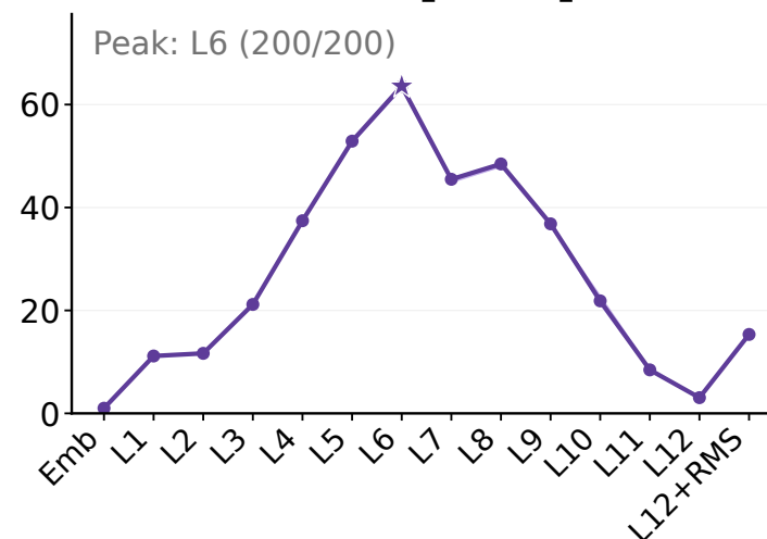
Uber [PT-ID]
