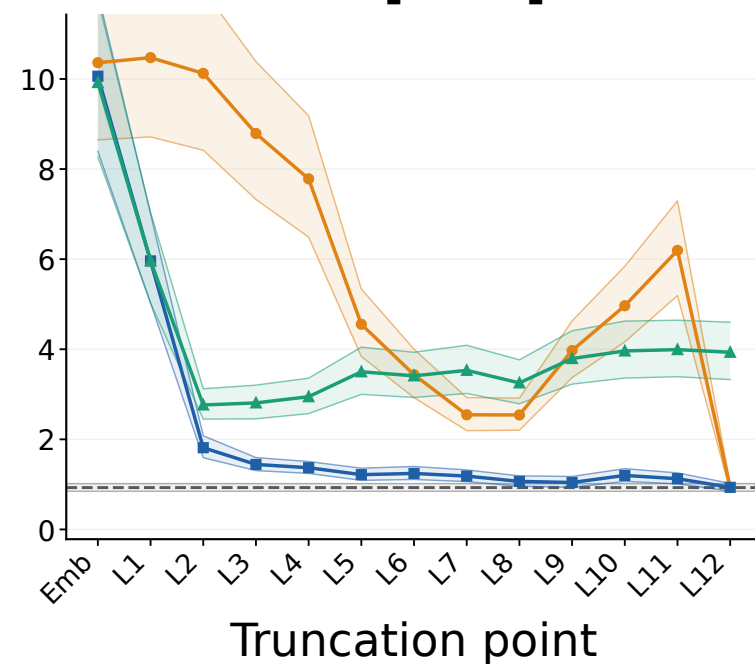
M4 [PT-ID]
