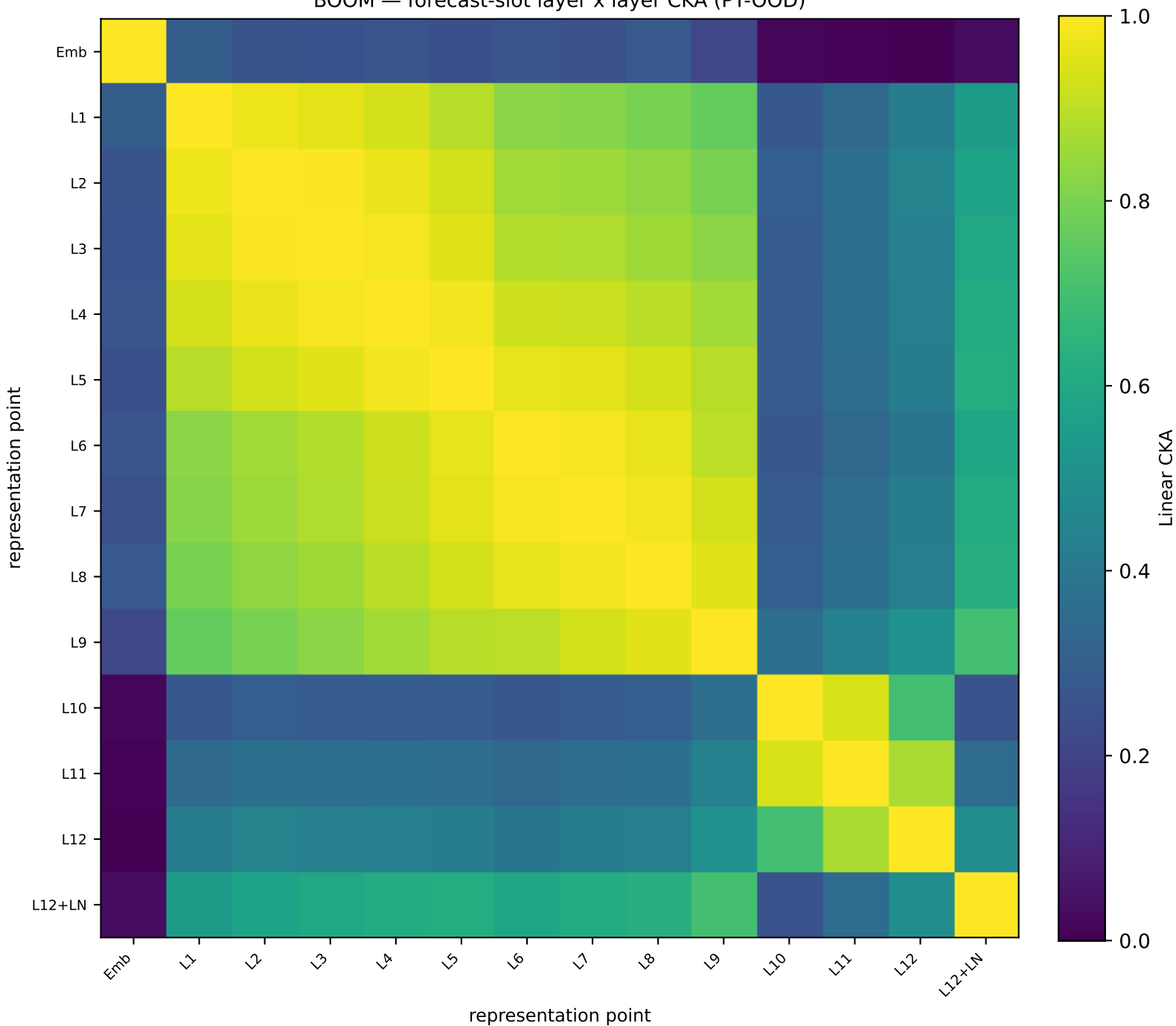
BOOM — forecast-slot layer x layer CKA (PT-OOD)
