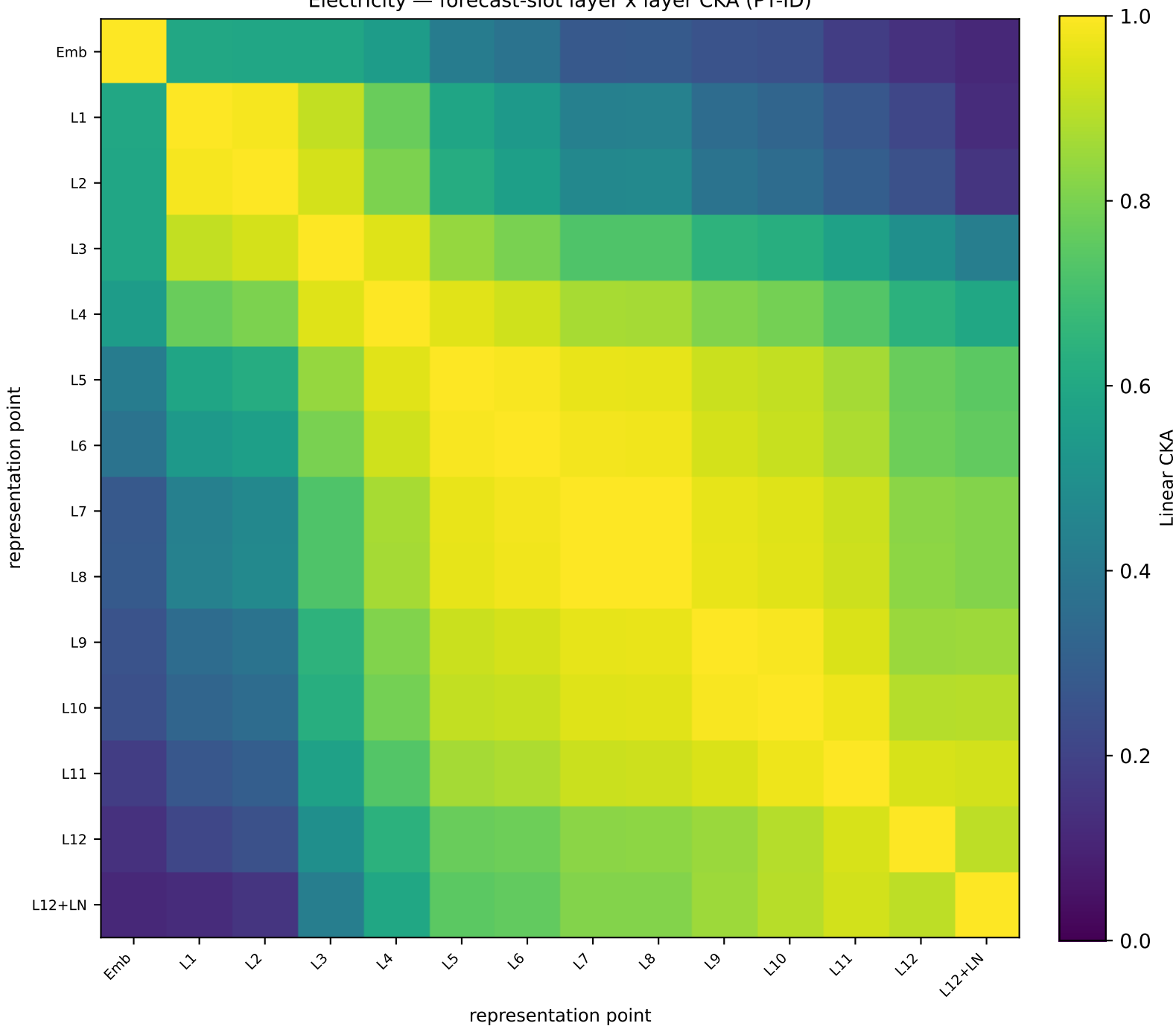
Electricity — forecast-slot layer x layer CKA (PT-ID)
