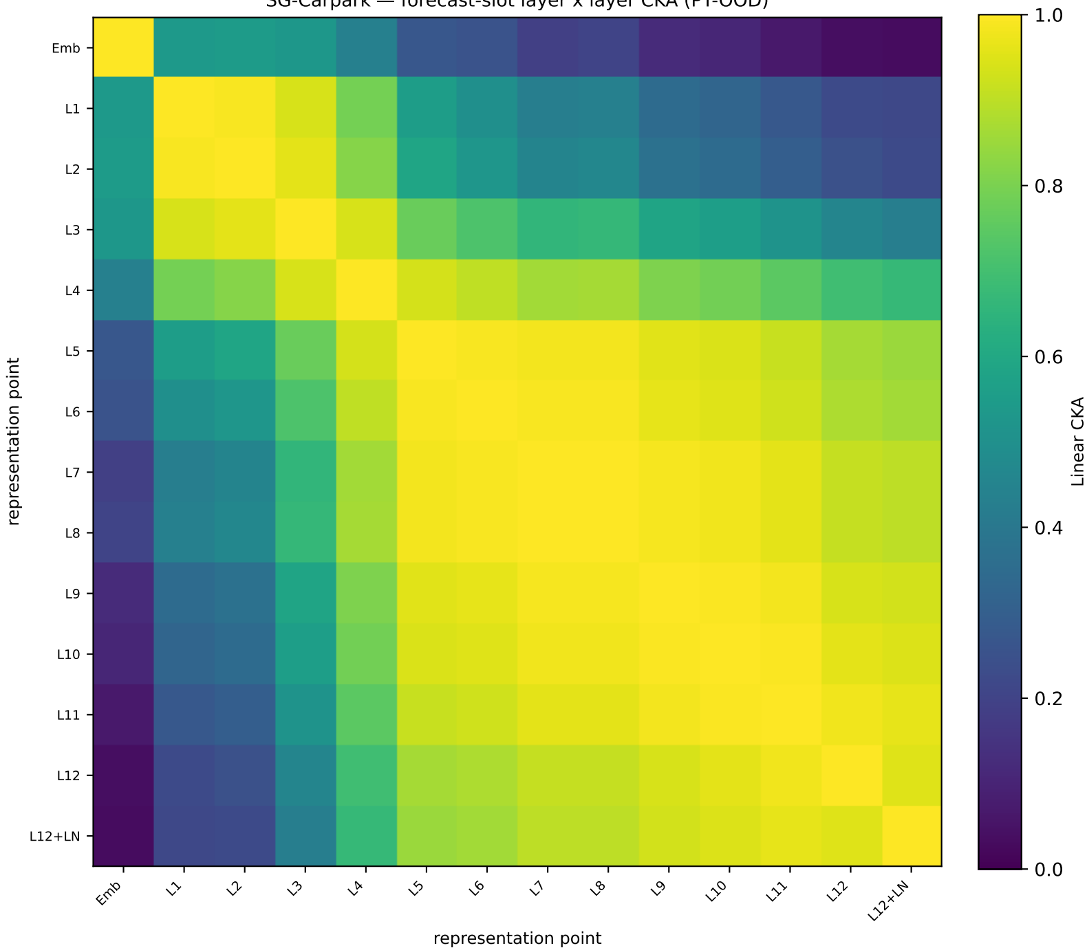
SG-Carpark — forecast-slot layer x layer CKA (PT-OOD)
