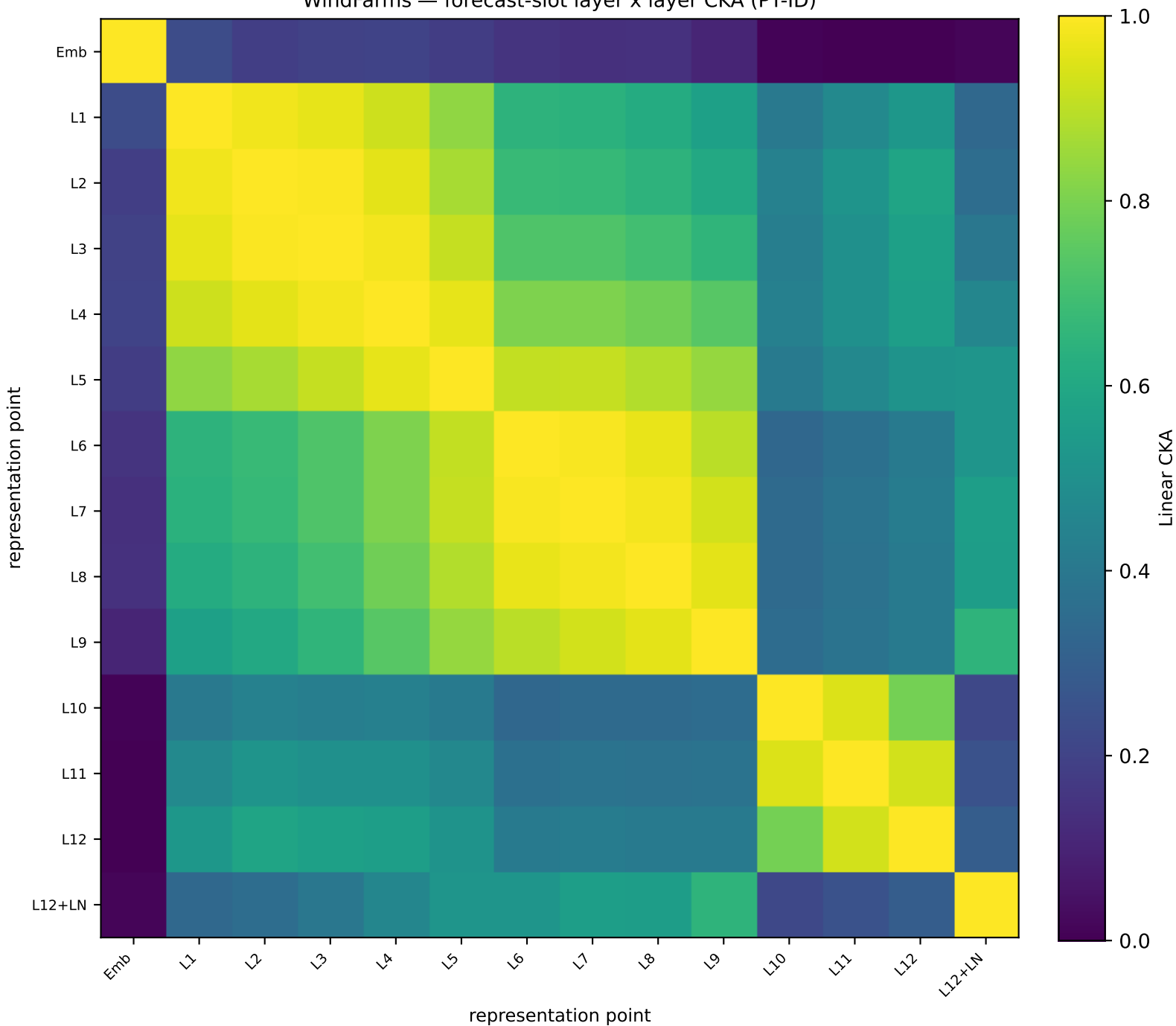
WindFarms — forecast-slot layer x layer CKA (PT-ID)
