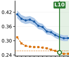
Uber TLC
