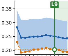
BOOM
