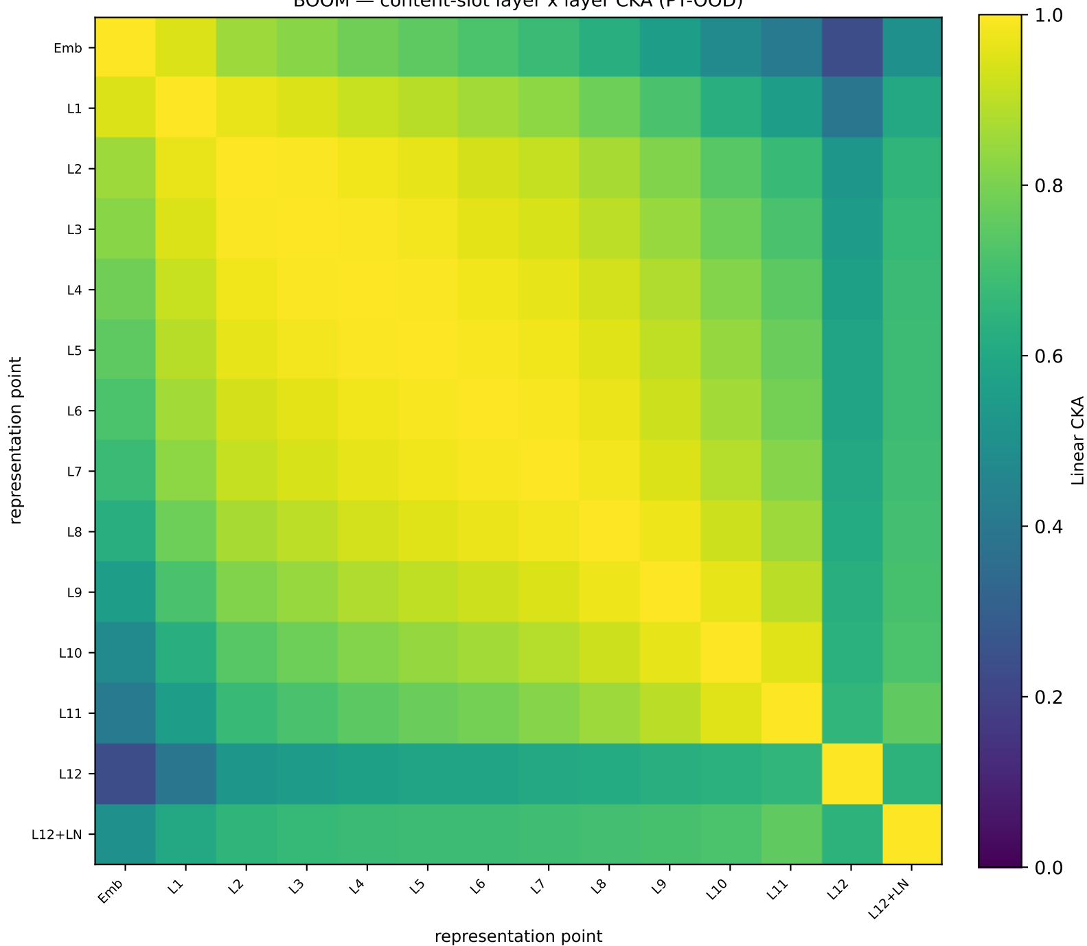
BOOM — content-slot layer x layer CKA (PT-OOD)
