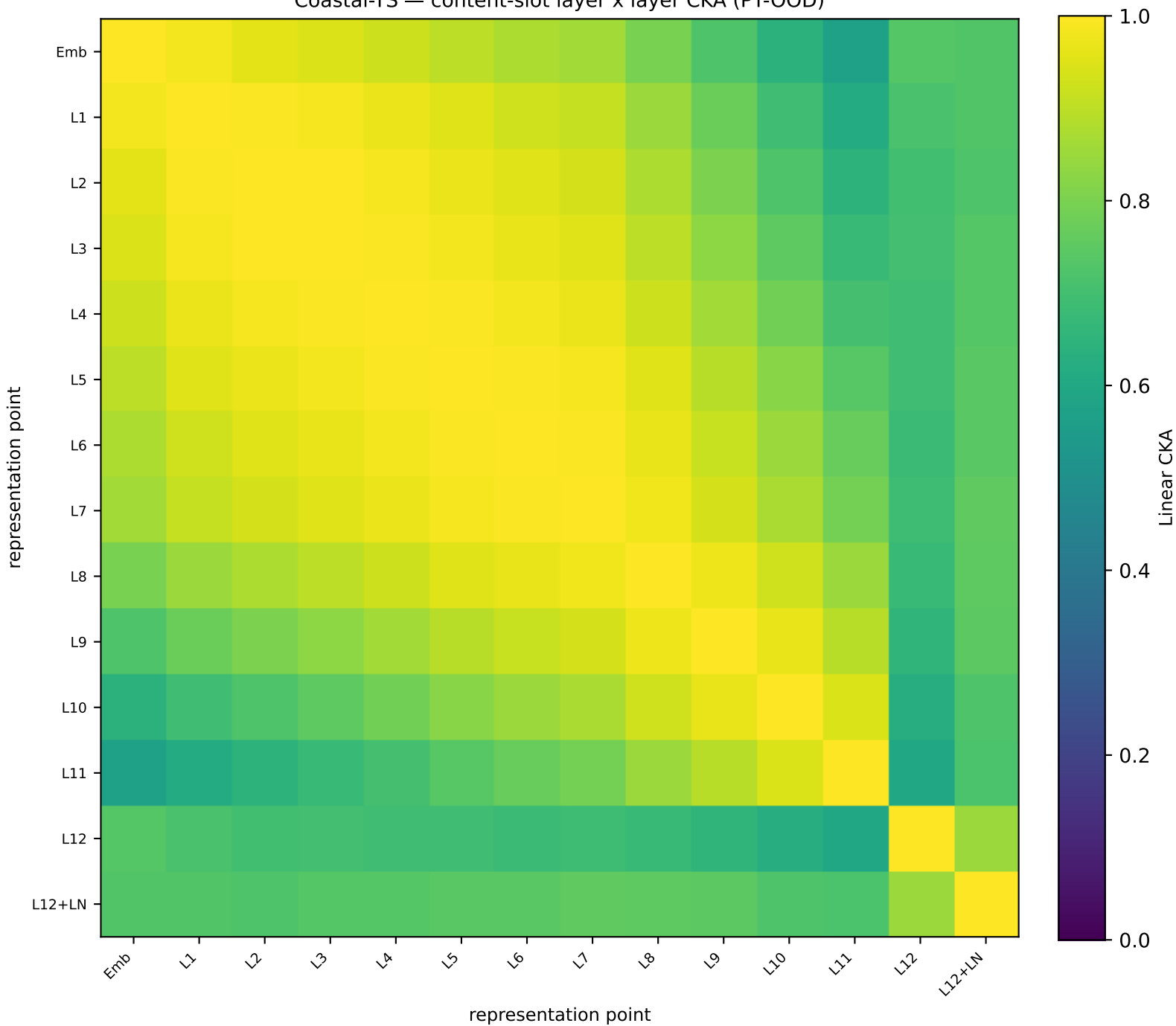
Coastal-TS — content-slot layer x layer CKA (PT-OOD)
