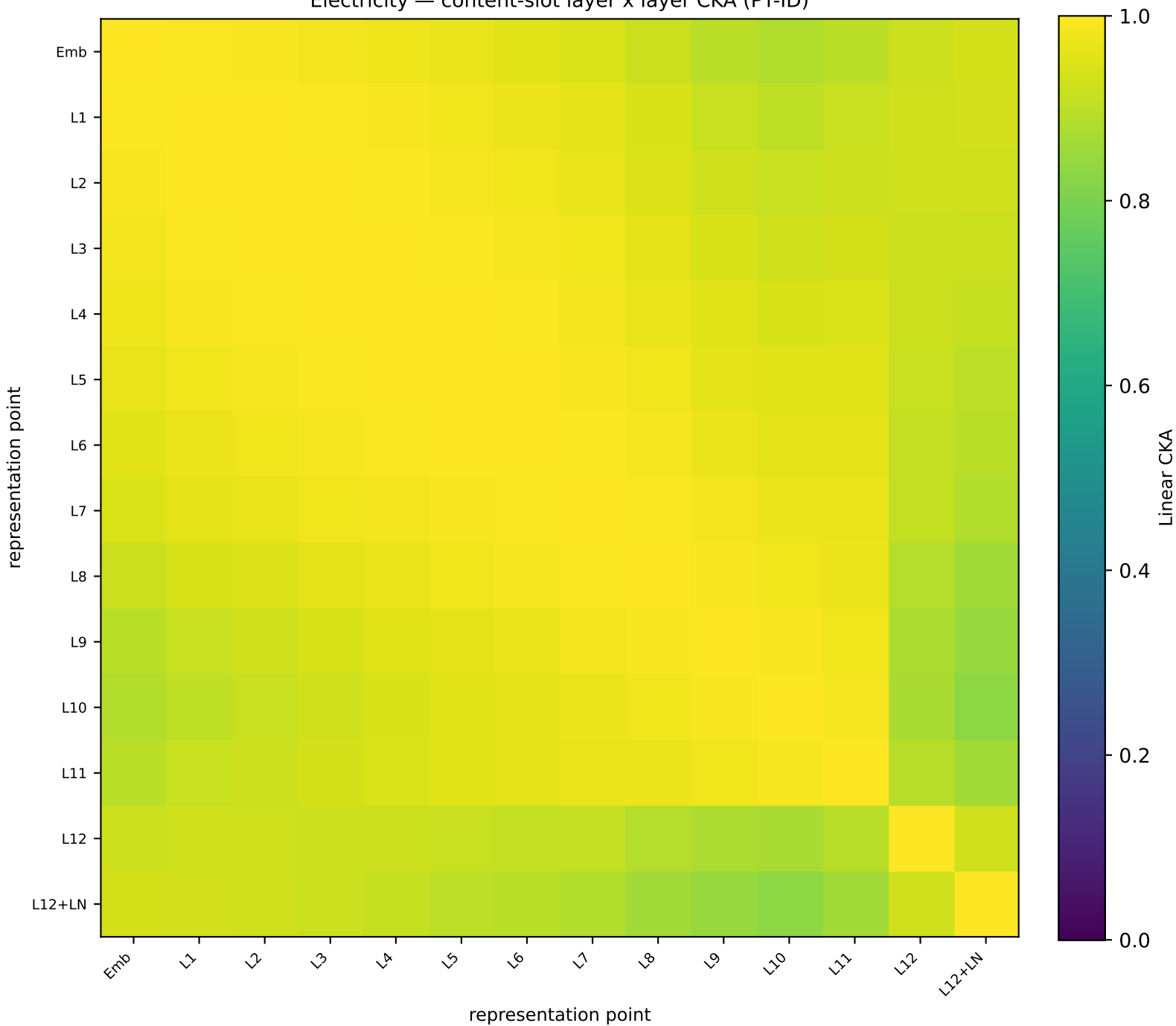
Electricity — content-slot layer x layer CKA (PT-ID)
