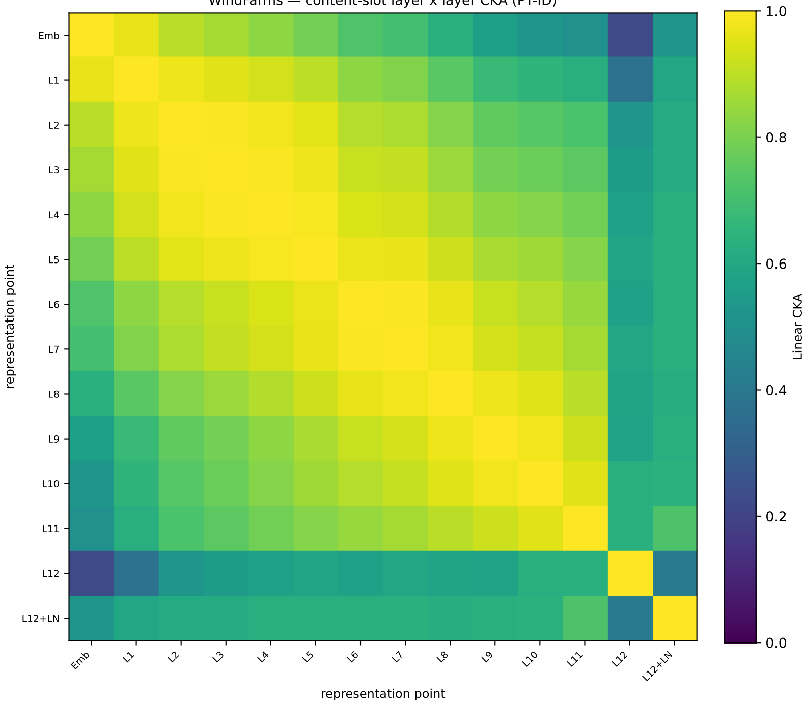
WindFarms — content-slot layer x layer CKA (PT-ID)
