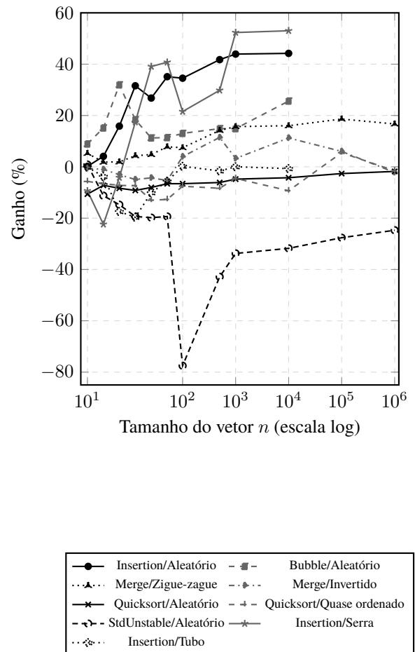
Figura 4. Ganho do pré-processamento em função do tamanho da entrada para pares algoritmo-topologia selecionados (mesmas médias do Criterion; métodos quadráticos limitados a n=10^5 ; lacunas são células não planejadas).
