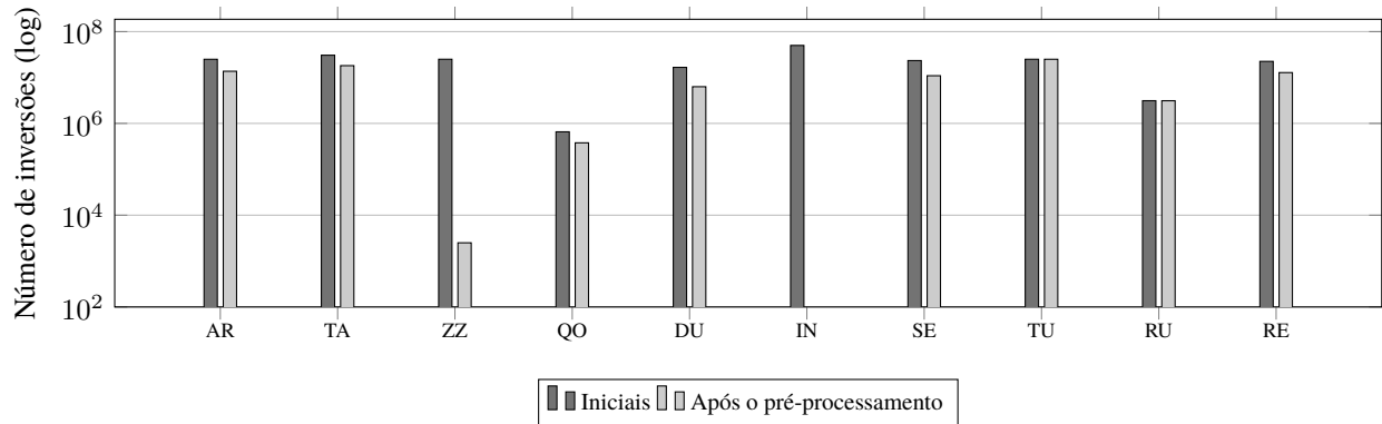
Figura 1. Número de inversões antes e após o pré-processamento simétrico para vetores de 10.000 elementos (escala logarítmica; no cenário Invertido o valor pós-pré-processamento é zero e não aparece na escala log). As abreviações são: AR (Aleatório), TA (Tartarugas), ZZ (Zigue-zague), QO (Quase ordenado), DU (Duplicados), IN (Invertido), SE (Serra), TU (Tubo), RU (Runs) e RE (Real).
