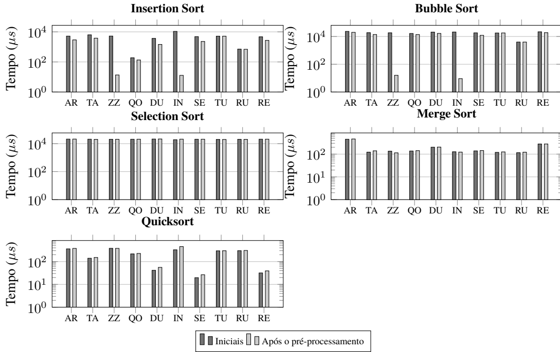
Figura 3. Comparação temporal entre a ordenação pura e com pré-processamento simétrico ( n = 10.000 ) nas dez topologias, em escala logarítmica. As abreviações são: AR (Aleatório), TA (Tartarugas), ZZ (Zigue-zague), QO (Quase ordenado), DU (Duplicados), IN (Invertido), SE (Serra), TU (Tubo), RU (Runs) e RE (Real).
