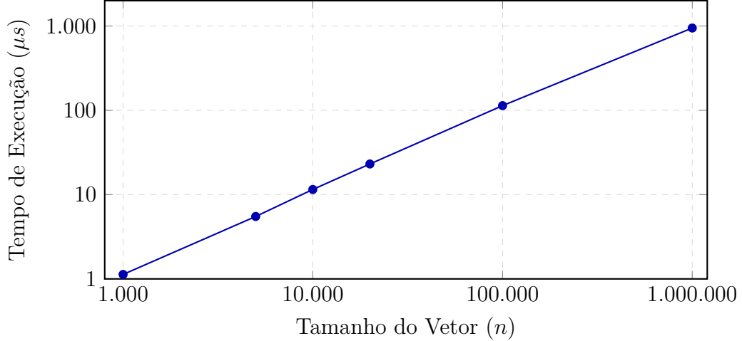
Figura 2. Tempo médio de execução do pré-processamento em função do tamanho do vetor ( n ), apresentado em escala log-log para evidenciar o comportamento linear O(n) . Valores médios sobre os dez tipos de entrada, obtidos pela ferramenta CLI com seed 42.
