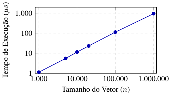
Figura 2. Tempo médio de execução do pré-processamento em função do tamanho do vetor ( n ), apresentado em escala log-log para evidenciar o comportamento linear O(n) . Valores médios sobre os dez tipos de entrada, obtidos pela ferramenta CLI com seed 42.
