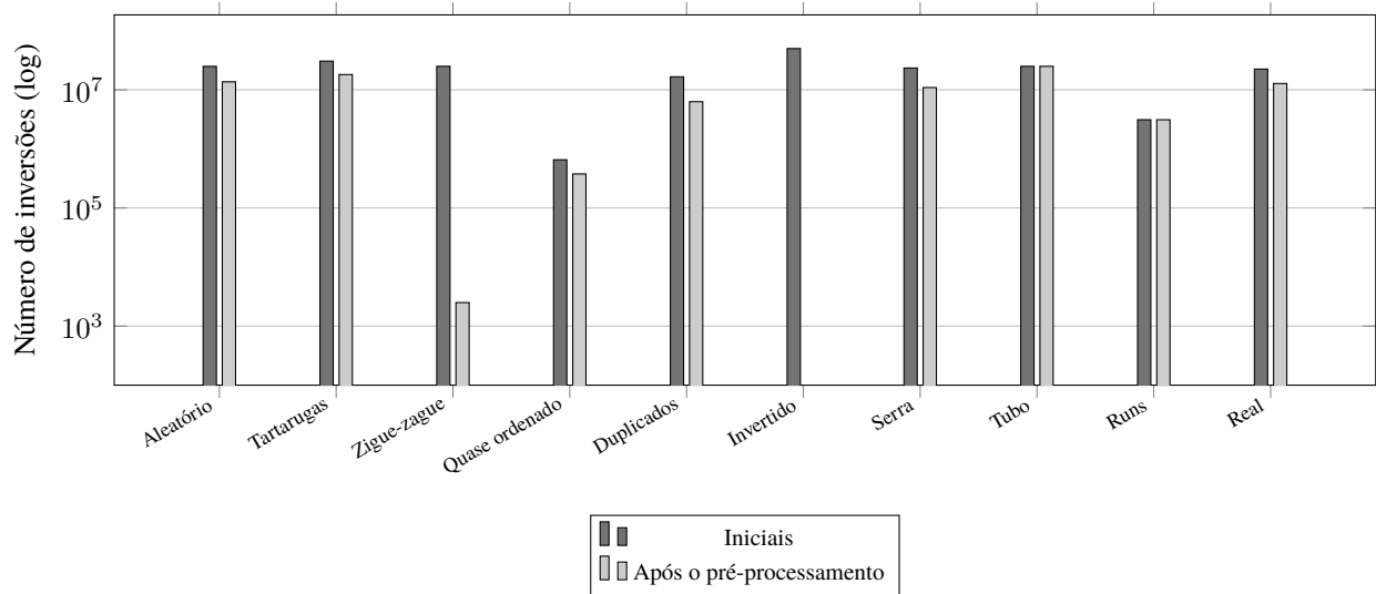
Figura 1. Número de inversões antes e após o pré-processamento simétrico para vetores de 10.000 elementos (escala logarítmica; no cenário Invertido o valor pós-pré é zero e não aparece na escala log).
