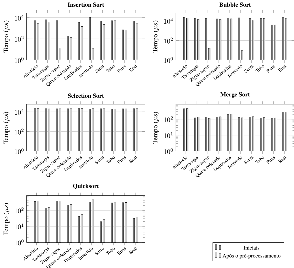
Figura 3. Comparação temporal entre a ordenação pura e com pré-processamento simétrico ( n = 10.000 ) nas dez topologias, em escala logarítmica.
