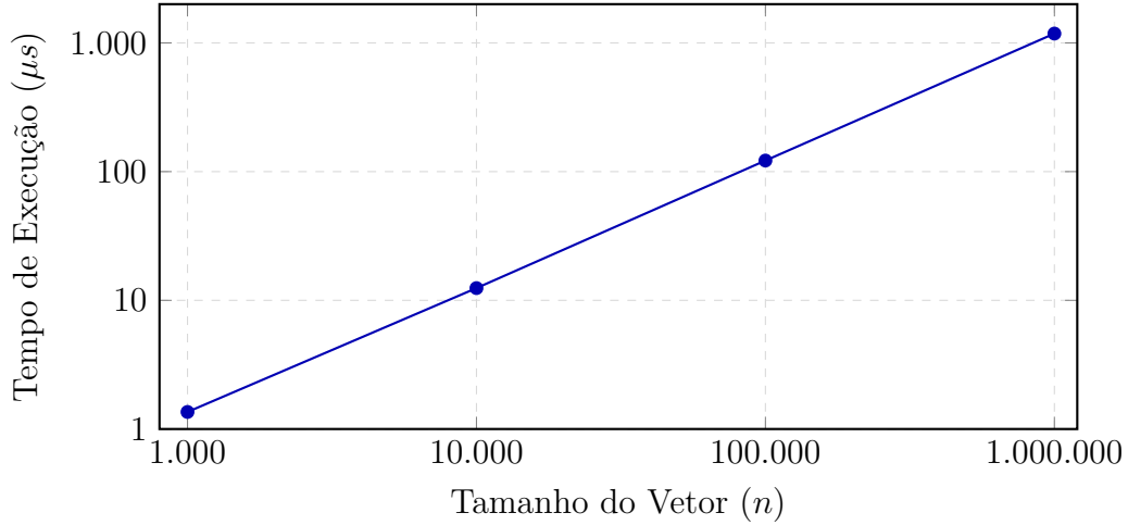
Figura 2. Tempo médio de execução do pré-processamento em função do tamanho do vetor ( n ), apresentado em escala log-log para evidenciar o comportamento linear O(n) . Valores médios sobre os seis tipos de entrada, obtidos pela ferramenta CLI com seed 42.
