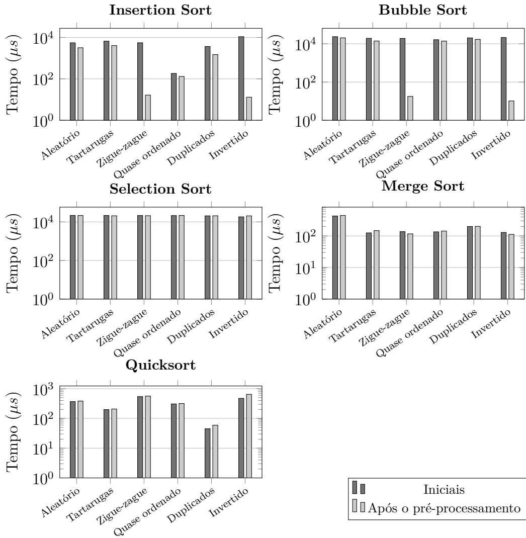
Figura 3. Comparação temporal entre a ordenação pura e com pré-processamento simétrico ( n = 10.000 ), em escala logarítmica.
