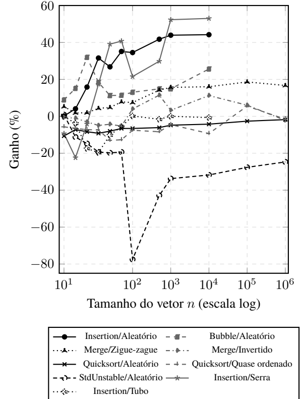
Figura 4. Ganho do pré-processamento em função do tamanho da entrada para pares algoritmo-topologia selecionados (mesmas médias do Criterion; métodos quadráticos limitados a n=10^5 ; lacunas são células não planejadas).
