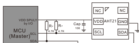
图15 典型应用电路1，SCL、SDA的上拉电压和VDD由MCU供电。
