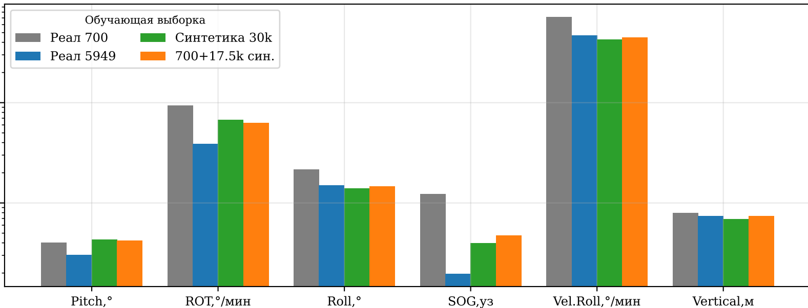
г) Ошибка по целям: объем реальных данных vs синтетика vs аугментация
