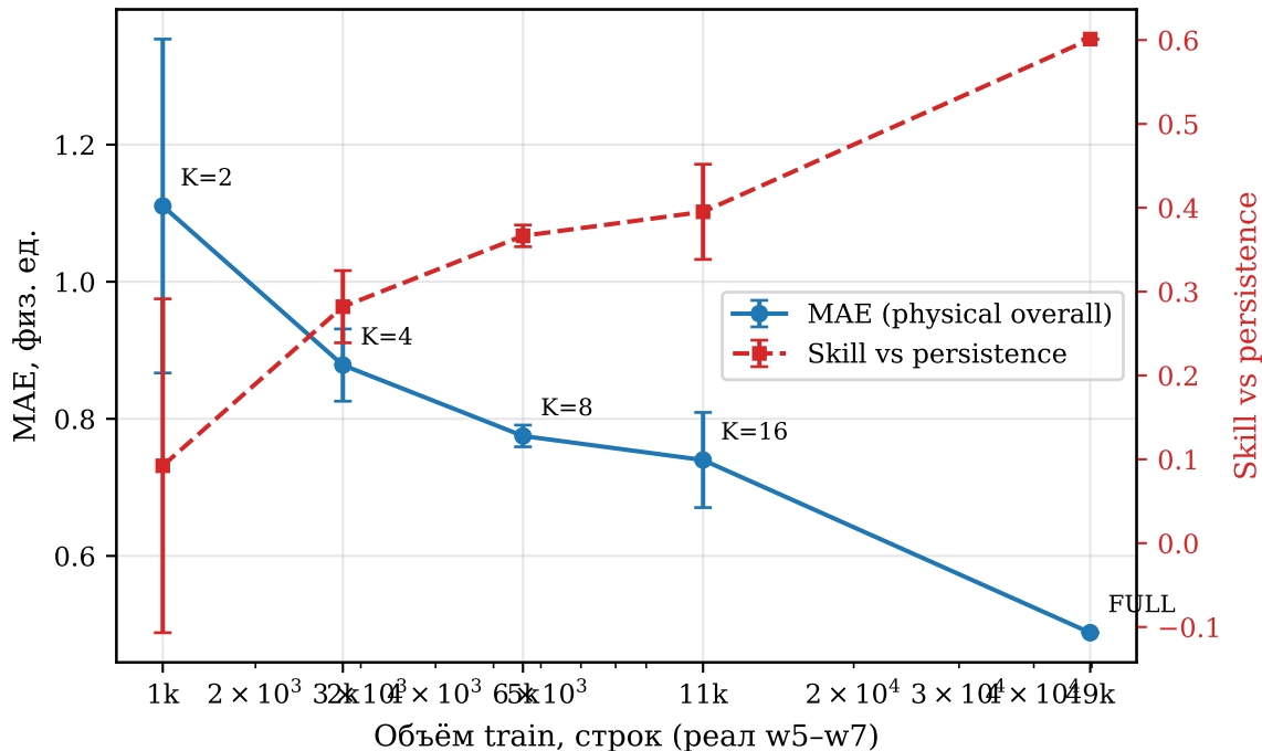
Learning curve на второй записи (E1T)
