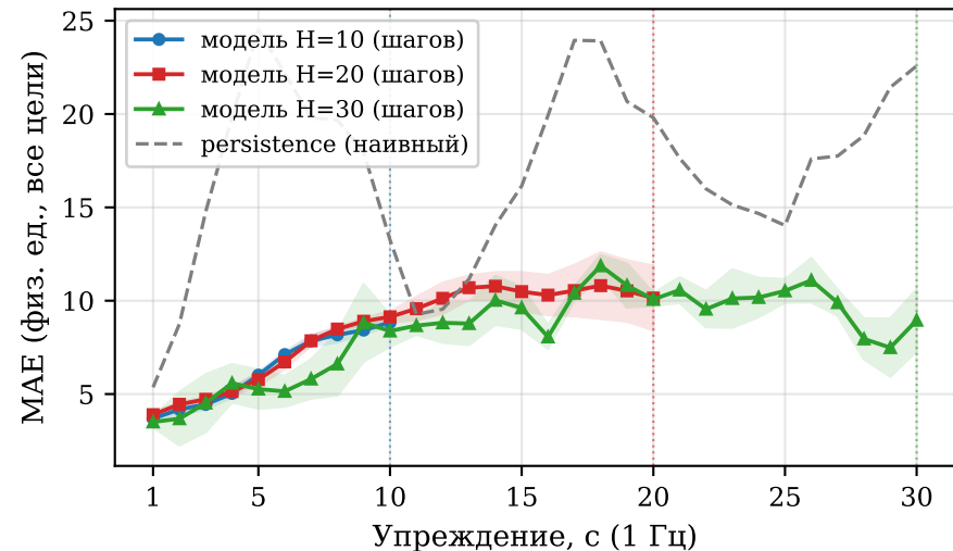
baseline (MSE + 0.5·Huber + 0.1·smooth, Roll=2)
