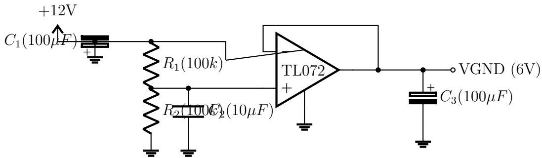
Figura 2.3: Schema electronică a sistemului de masă virtuală.
