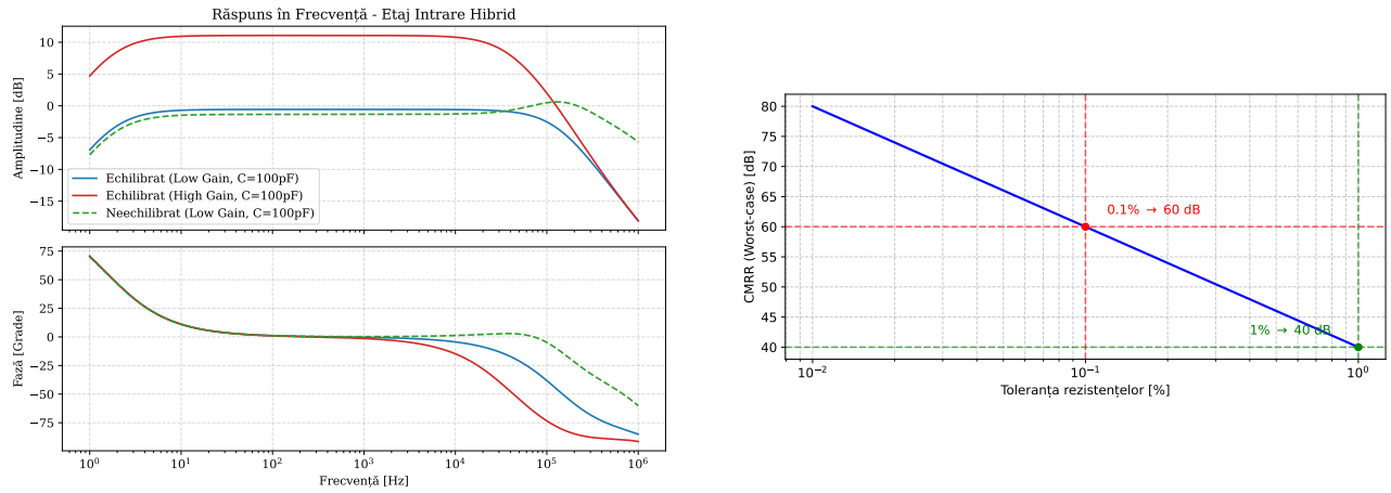
Figura 2.3: Analiza performanțelor interfeței de intrare prin simulare numerică. (Stânga) Răspunsul plat în banda audio pentru diferite moduri de operare. (Dreapta) Eficiența rejecției modului comun în funcție de toleranța rezistențelor.
