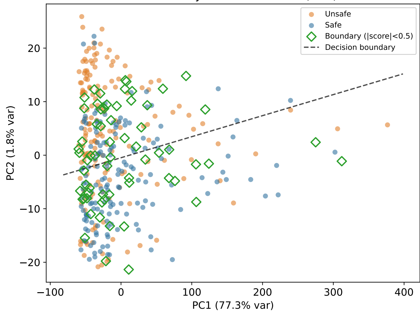
IT-Model Layer 10 Activations (PCA)
