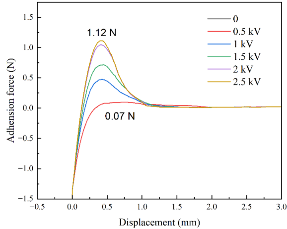
图 1.8 VSERF 粘附力随电压变化曲线
