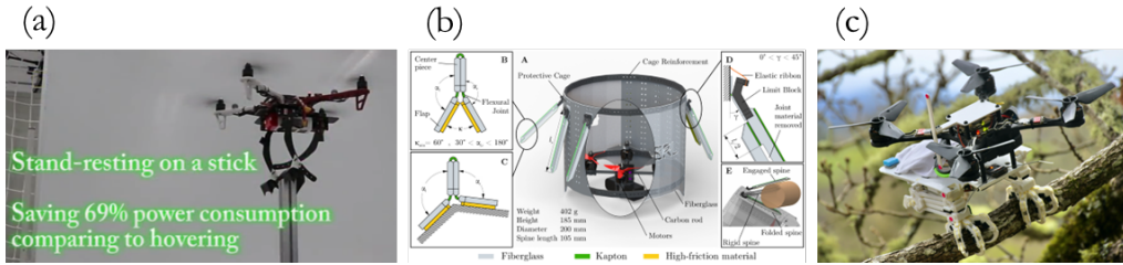
图 1.2 部分基于抓握的栖息无人机设计，(a) [2] , (b) [2] , (c) [2]
