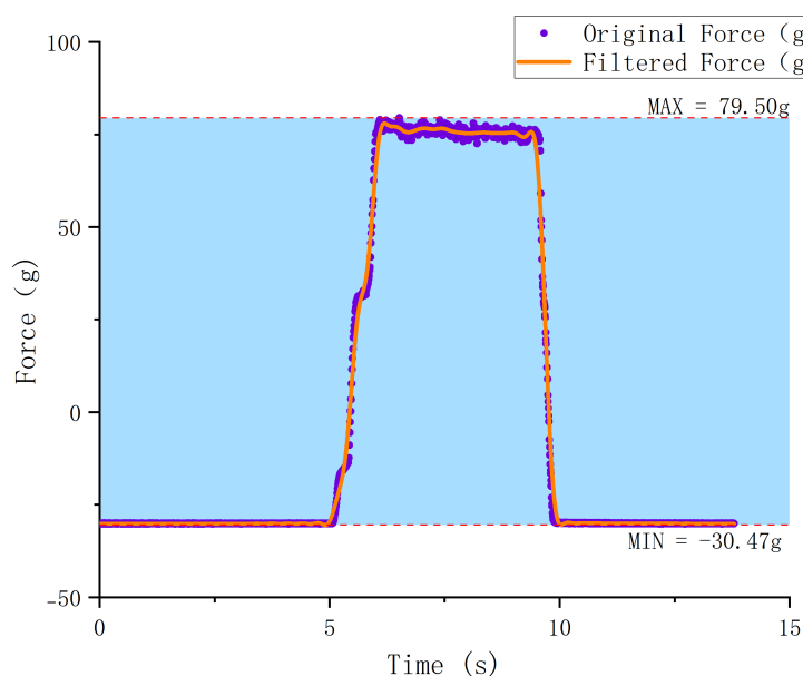
图 1.12 全油门推力测试图
