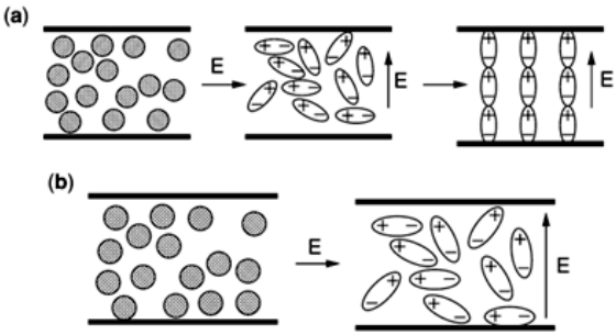
图 1.4 电流变液（ERF）机理解释。(a) ER 粒子，(b) 非 ER 粒子 [2]
