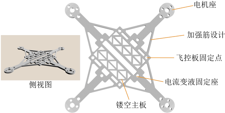
图 1.9 无人机底座设计图
