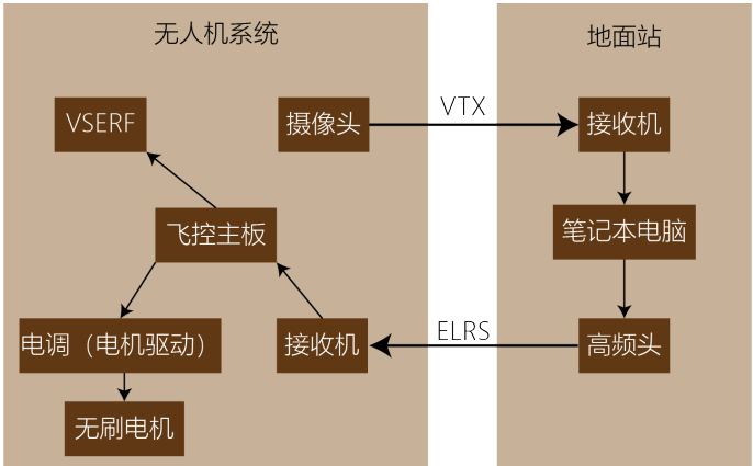
图 1.10 系统通信设计
