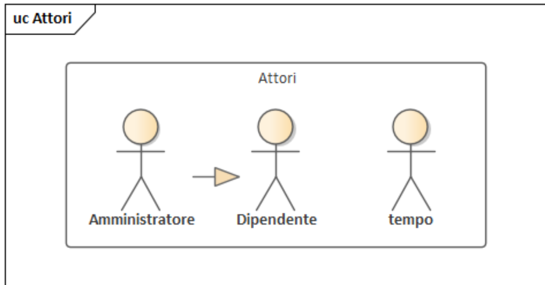
Figura 3: Schematizzazione degli attori
