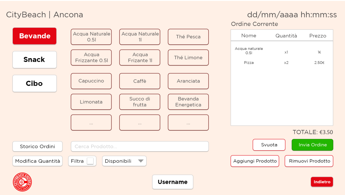
Figura 39: Schermata Area Ristoro
