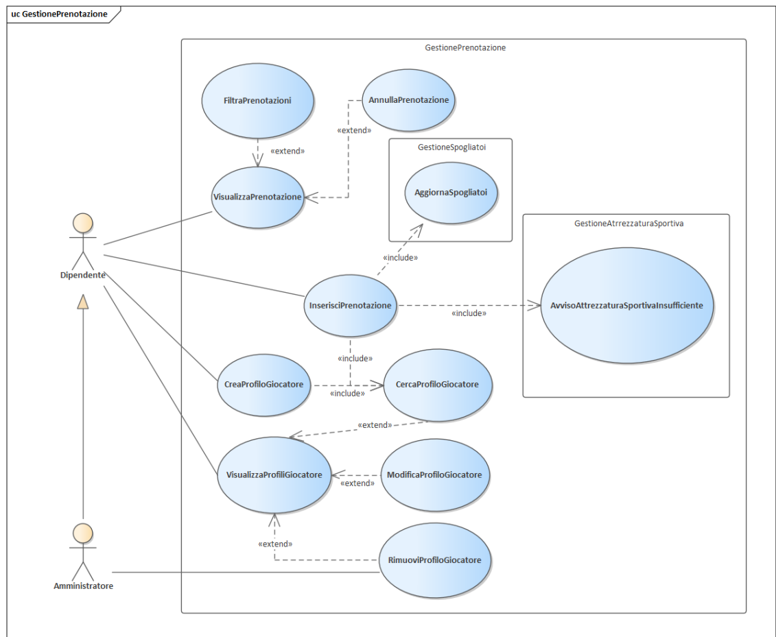
Figura 5: Diagramma Gestione Prenotazione
