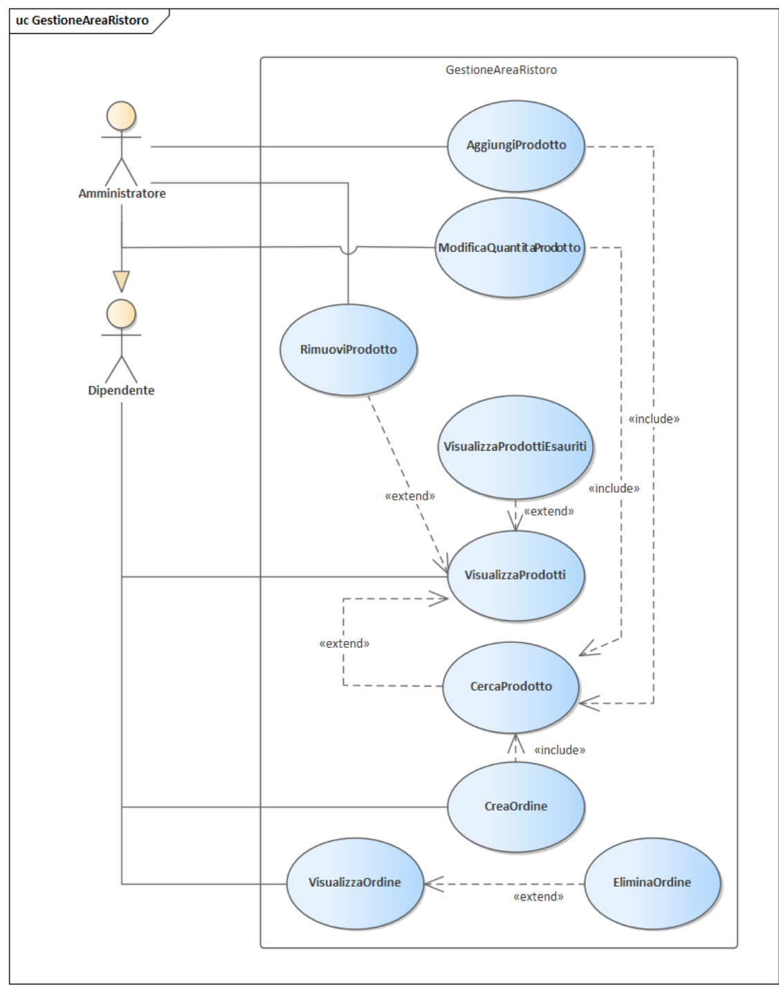
Figura 8: Diagramma Gestione Area Ristoro
