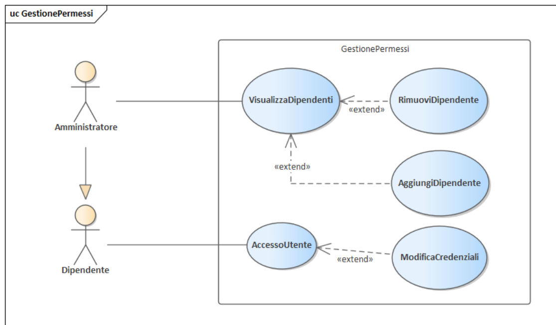
Figura 9: Diagramma Gestione Permessi
