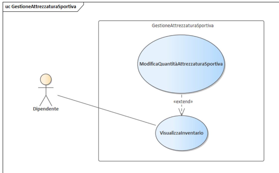
Figura 6: Diagramma Gestione Attrezzatura Sportiva
