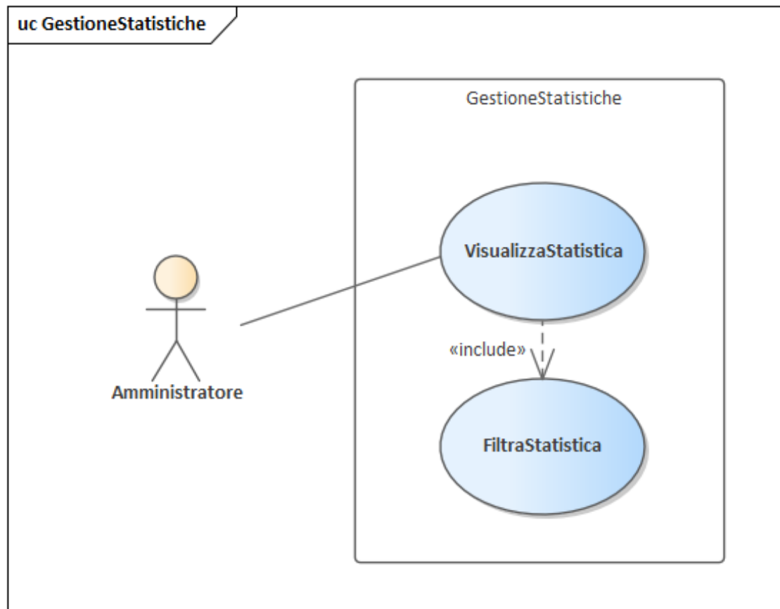
Figura 10: Diagramma Gestione Statistiche
