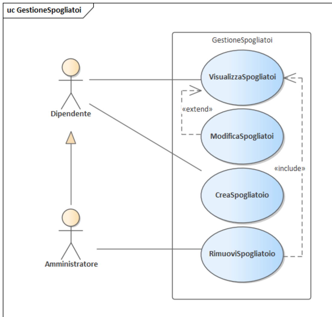
Figura 7: Diagramma Gestione Spogliatoi
