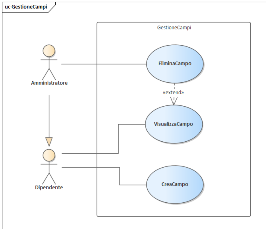
Figura 4: Diagramma Gestione Campi
