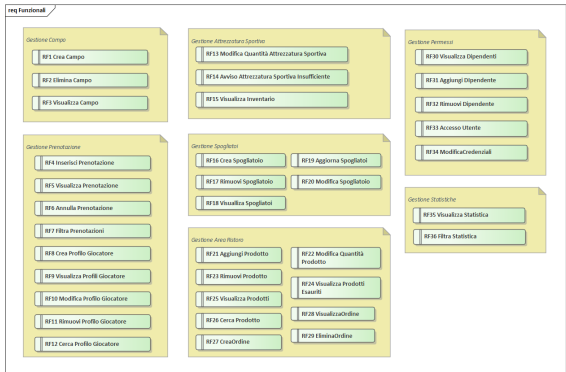
Figura 1: Schematizzazione dei requisiti Funzionali
