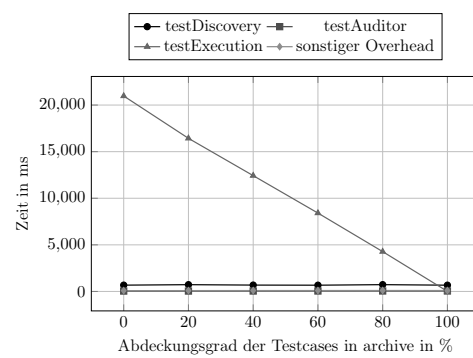
(f) viele langsame Testcases: T=10.000, I=10.000.000
