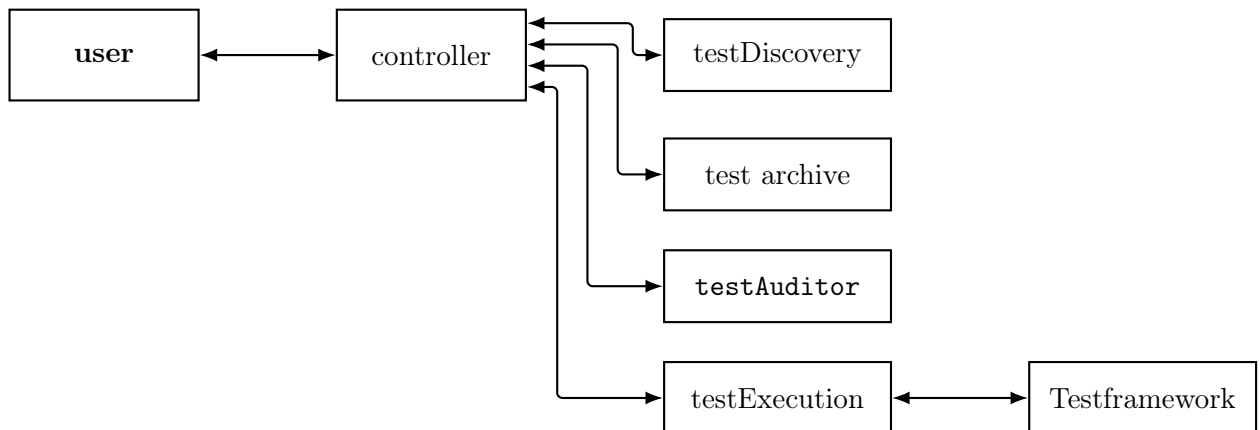
Abbildung 1: Schematische Darstellung der Interaktion von user , controller , testAuditor , Hilfskomponenten und dem Testframework.
