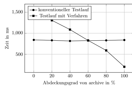
(d) viele mittellange Testcases: T=1000 , I=10000
