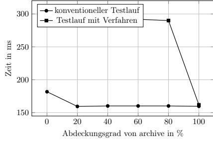
(a) wenige kurze Testcases: T=10 , I=100
