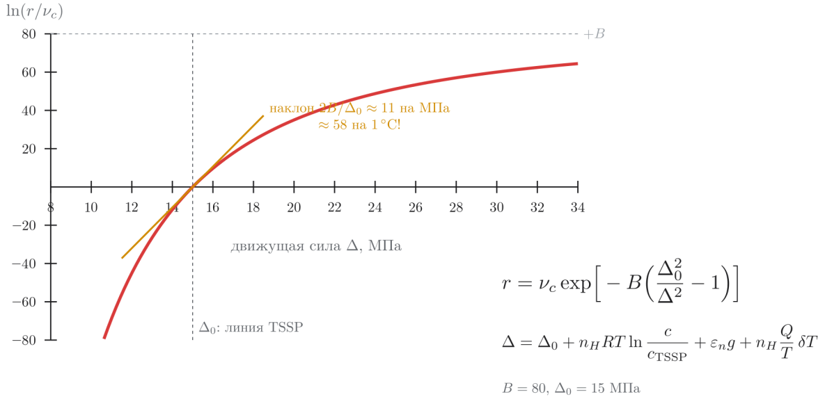
Рис. 5.2: Логарифм скорости зарождения от движущей силы. У линии TSSP ( \Delta = \Delta_0 ) кривая очень крутая: +1 МПа — скорость больше в e^{11} раз, +1 °C — в e^{58} .
