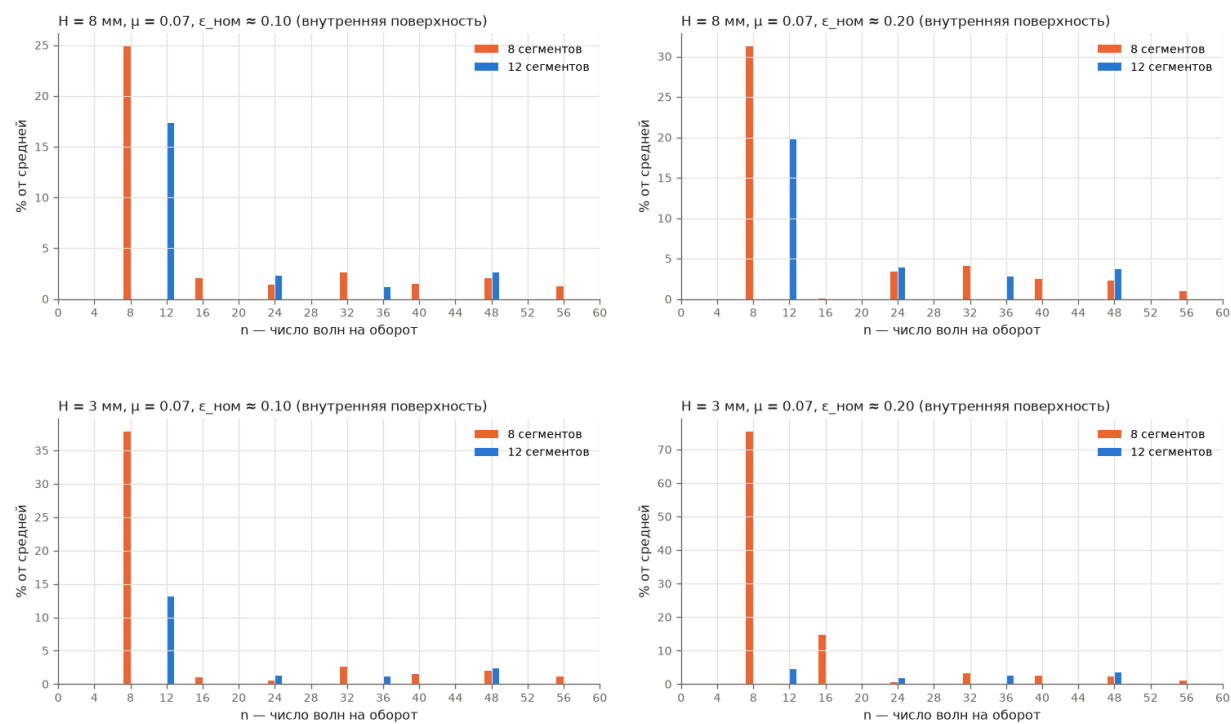
Рис. 6. Спектры деформации внутренней поверхности для 8 и 12 сегментов (секторные модели, \mu = 0.07 ) при \epsilon_{\text{ном}} \approx 0.10 и 0.20 . Высота столбика — в процентах от средней деформации.
