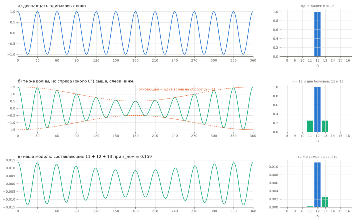
Рис. 4. а) Двенадцать одинаковых волн — в спектре одна линия n = 12 . б) Те же волны, но выше справа и ниже слева (оггибающая — одна волна на оборот): в спектре появляются две боковые линии, n = 11 и n = 13 . в) То же в нашей модели (составляющие 11 + 12 + 13 ): волны сегментов на тонкой стороне (около 0^\circ ) выше, чем на толстой (около 180^\circ ).
