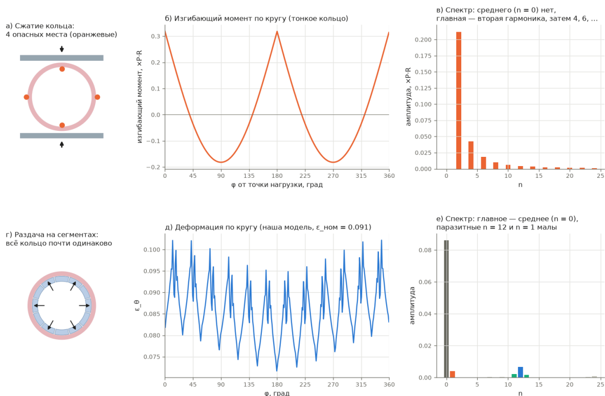
Рис. 8. Сверху — сжатие кольца: изгибающий момент по кругу (формула для тонкого кольца) и его спектр. Снизу — раздача на сегментах: деформация по кругу (наша модель) и её спектр.
