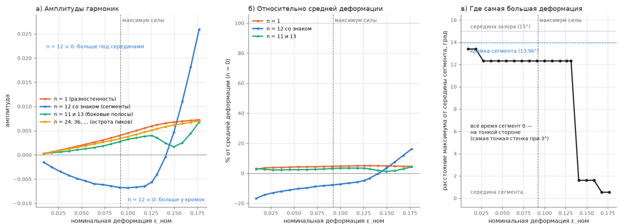
Рис. 5. Модель всего кольца ( H = 3 мм, 12 сегментов, \mu = 0.05 , разностенность \pm 1\% ), расчёт ещё идёт — показано до \epsilon_{\text{ном}} = 0.177 . а) Амплитуды; волна сегментов показана со знаком: «-» — деформация больше у кромок, «+» — под серединами сегментов. б) Те же амплитуды в процентах от средней деформации. в) Где самая большая деформация — расстояние от середины сегмента.
