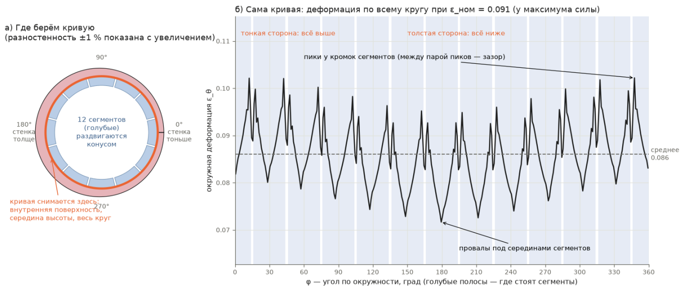
Рис. 1. а) Кривая снимается по внутренней поверхности посередине высоты; стенка чуть тоньше справа ( \phi \approx 0^\circ ) и толще слева ( 180^\circ ), разница \pm 1\% (на схеме увеличена). б) Деформация по кругу при номинальной деформации \epsilon_{\text{ном}} = 0.091 , у максимума силы. Голубые полосы — где стоят сегменты.
