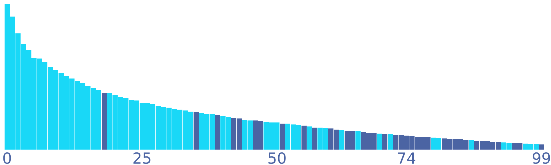
Layer 30
