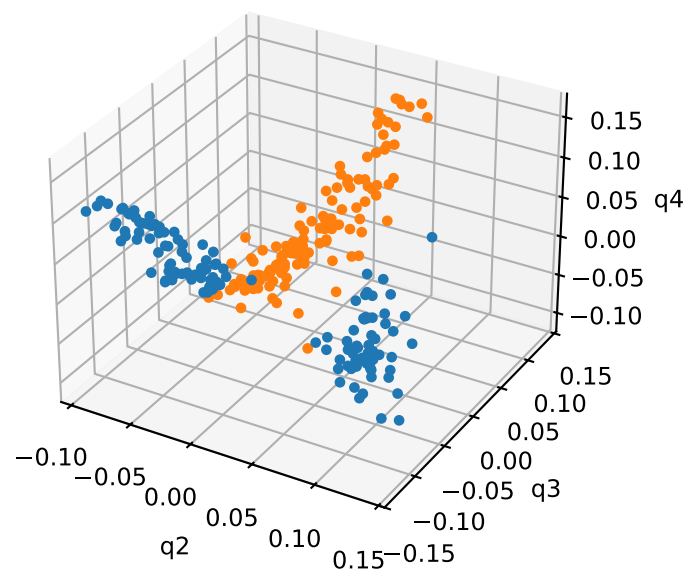
E-5: invariant subspace (q2,q3,q4)
