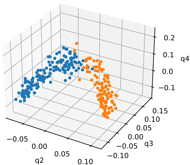
E-5: invariant subspace (q2,q3,q4)
