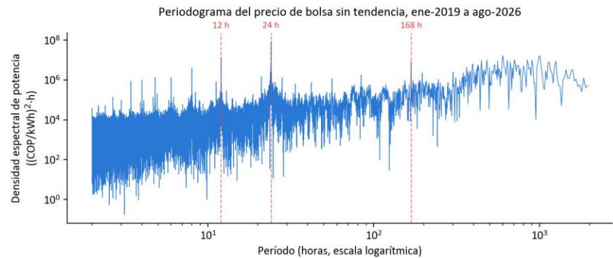
Figura 4. Periodograma del precio de bolsa sin tendencia. Líneas rojas: períodos de 12, 24 y 168 h.
