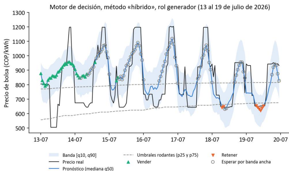
Figura 7. Motor de decisión en operación, método «híbrido» para el generador (13 al 19 de julio de 2026): pronóstico mediano, banda [q_{10}, q_{90}] , umbrales rodantes y acción recomendada en cada hora.
