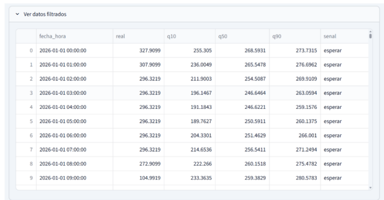
Figura 9. Detalle de la vista Analista: (a) selección manual del método de umbral; (b) datos filtrados hora por hora con el precio real, los cuantiles del pronóstico y la señal del motor.
