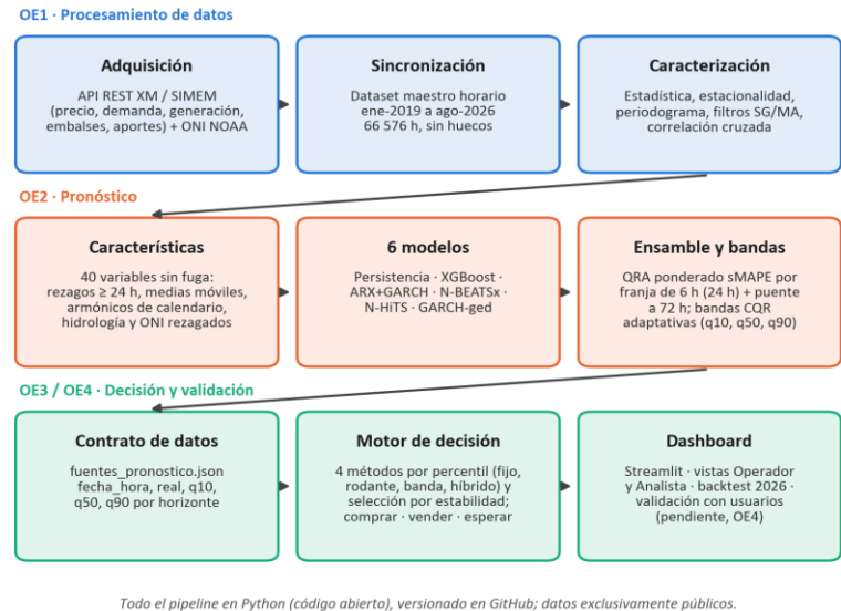
Figura 2. Diagrama de bloques de la plataforma y su relación con los objetivos específicos. Fuente: elaboración propia.
