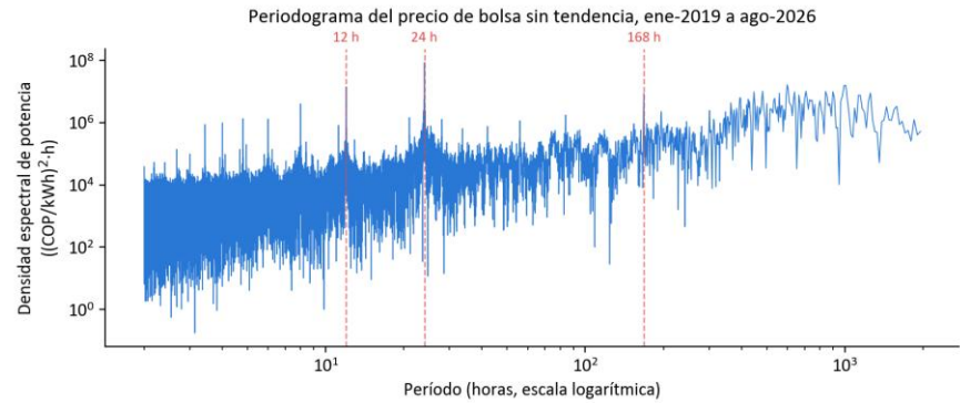
Figura 10. Periodograma del precio de bolsa sin tendencia. Líneas rojas: períodos de 12, 24 y 168 h.
