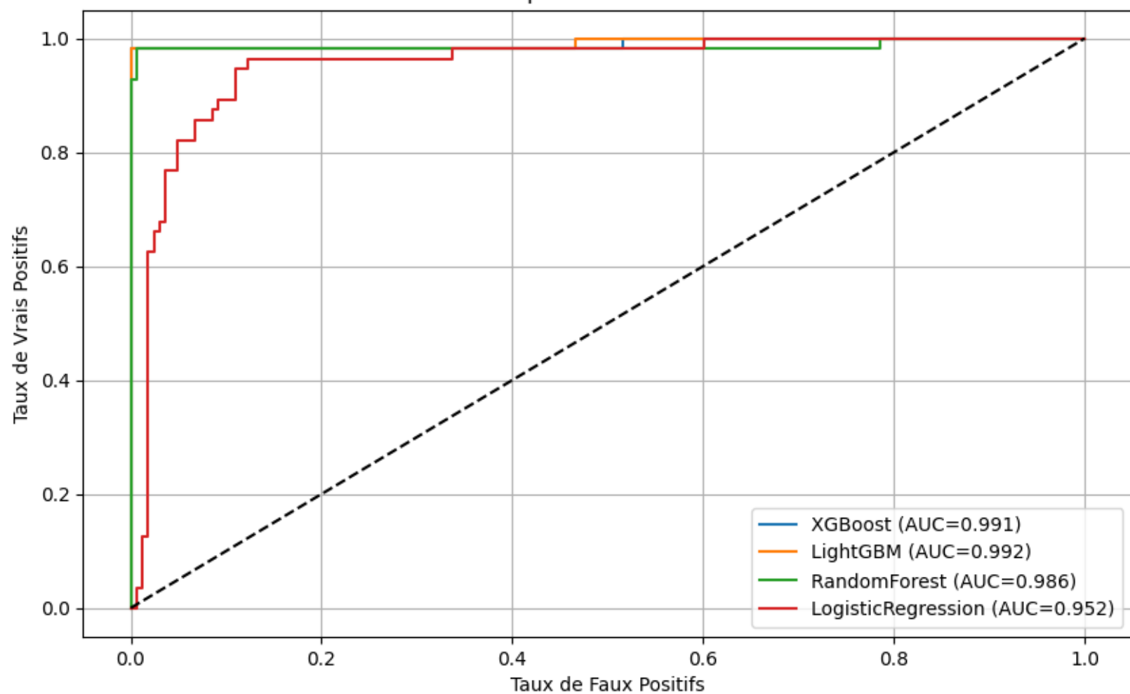
Courbes ROC - Comparaison des modèles BRCA TCGA
