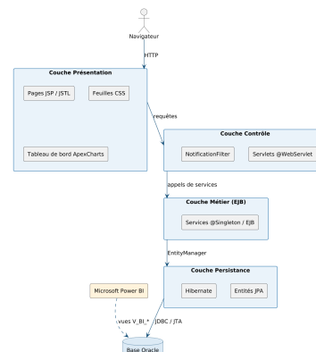
Architecture logique en couches
