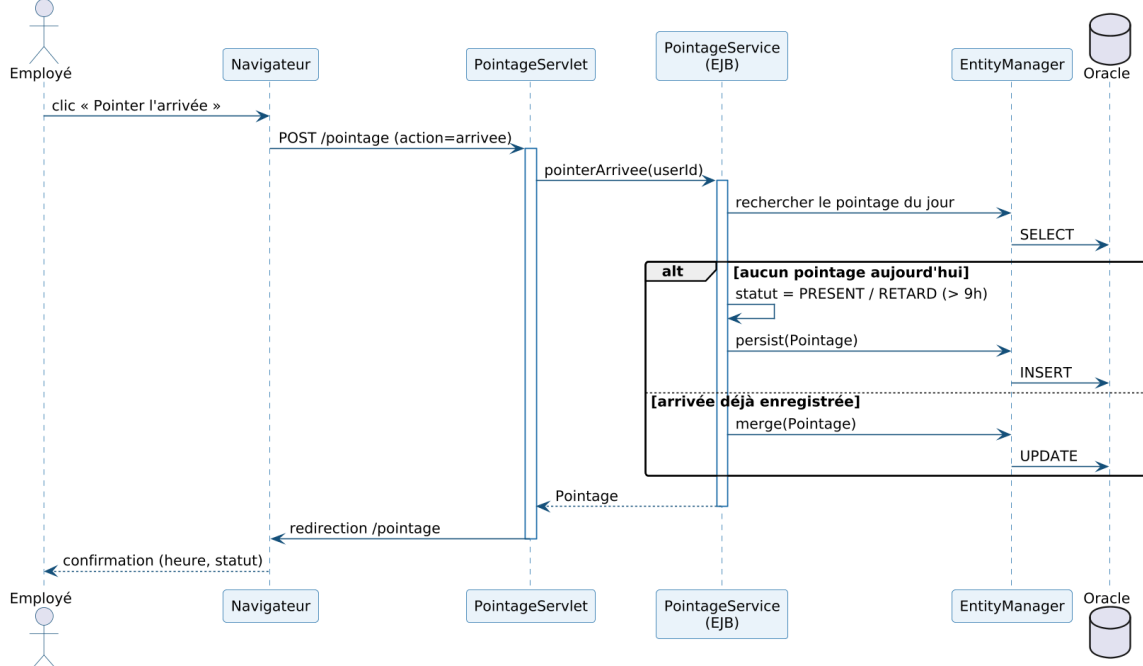
FIGURE 6.2 – Diagramme de séquence – Pointage d'un employé
