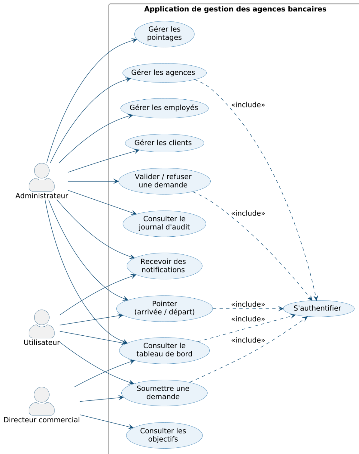
FIGURE 2.1 – Diagramme de cas d'utilisation global
