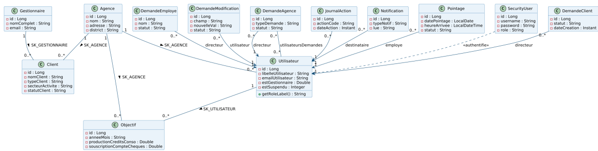
FIGURE 2.2 – Diagramme de classes du modèle métier
