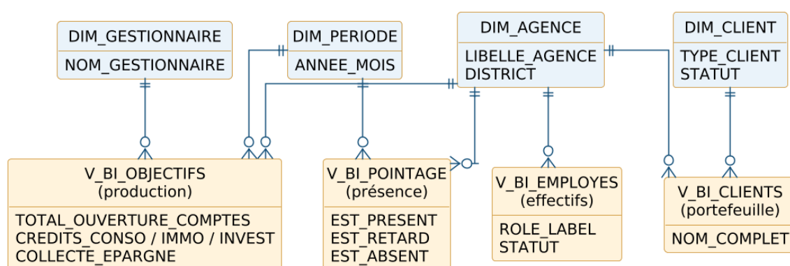
FIGURE 7.3 – Modèle décisionnel en étoile (vues V_BI_*)
