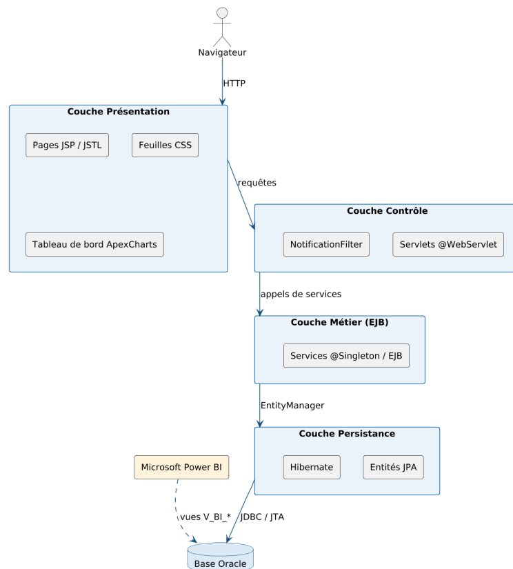
FIGURE 2.18 – Architecture logique en couches de l'application
