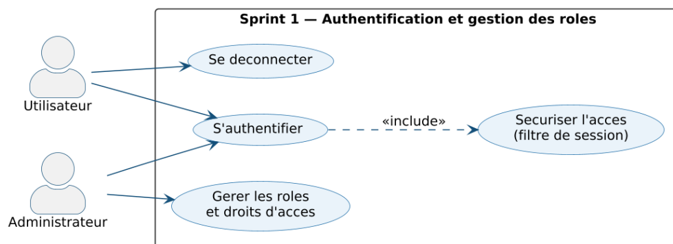
FIGURE 3.1 – Diagramme de cas d'utilisation du Sprint 1
