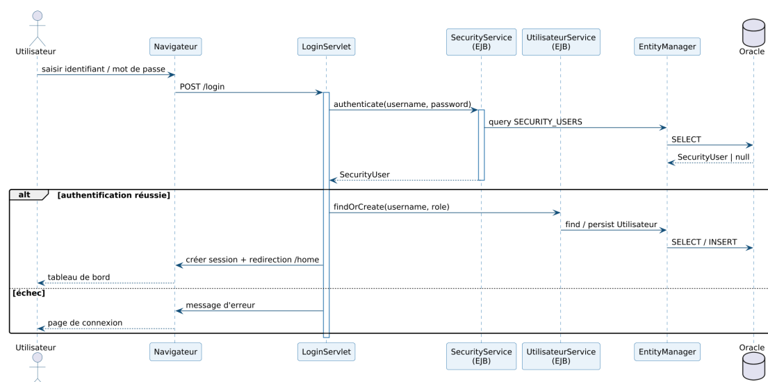
FIGURE 3.2 – Diagramme de séquence – Authentification
