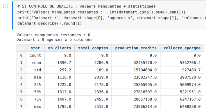
Figure 4.5 – Contrôle de qualité : statistiques du datamart (données réelles du réseau BTK)
