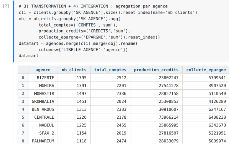
Figure 4.4 – Datamart par agence sur les données réelles du réseau BTK (portefeuille et production)
