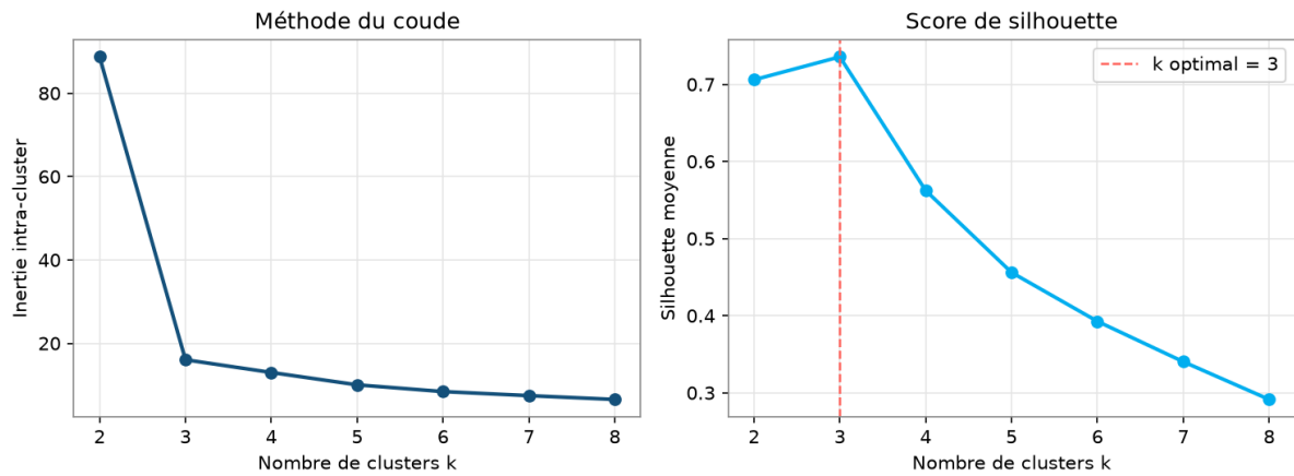
Figure 4.8 – Choix du nombre de clusters : méthode du coude et score de silhouette
