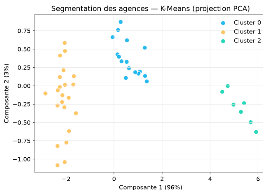
Figure 4.10 – Segmentation des agences (K-Means) projetée par PCA
