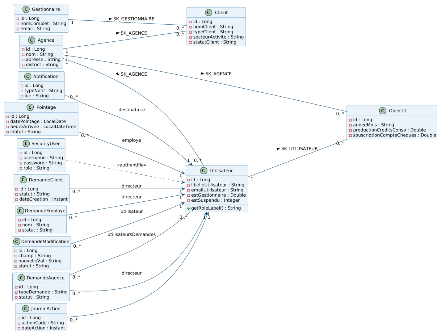
FIGURE 2.2 – Diagramme de classes du modèle métier
