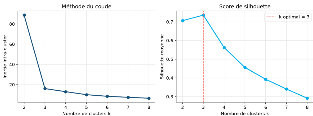
Figure 4.11 – Choix du nombre de clusters : méthode du coude et score de silhouette
