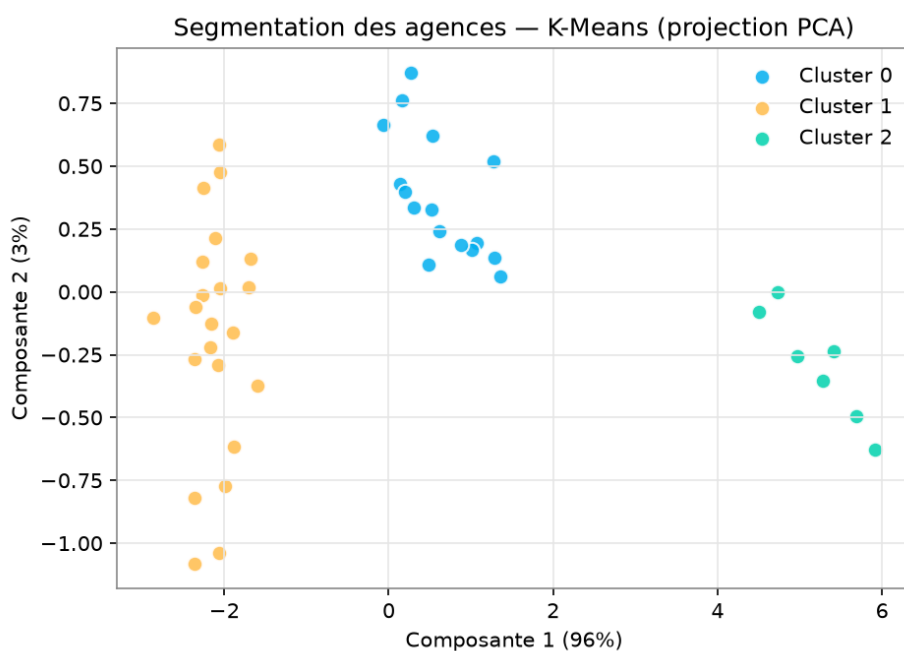
Figure 4.13 – Segmentation des agences (K-Means) projetée par PCA
