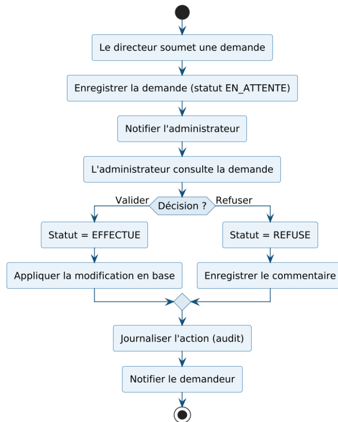
Figure 3.12 – Diagramme d'activité – Traitement d'une demande
