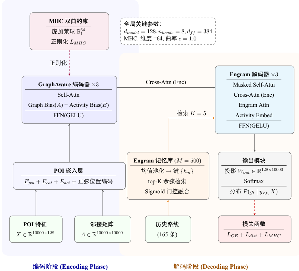
图 1 RouteTransformer 旅游路线生成模型架构图
