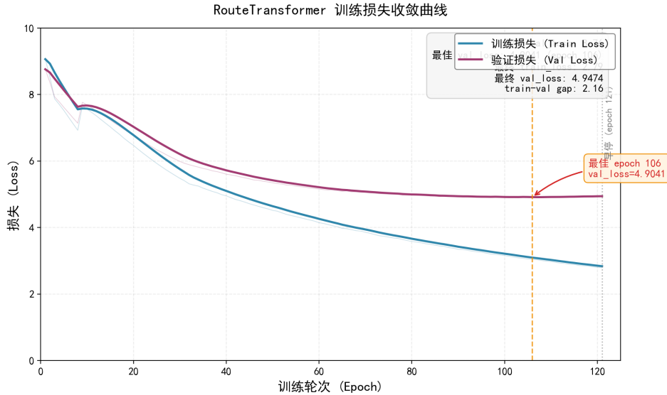
图 2 训练损失收敛曲线
