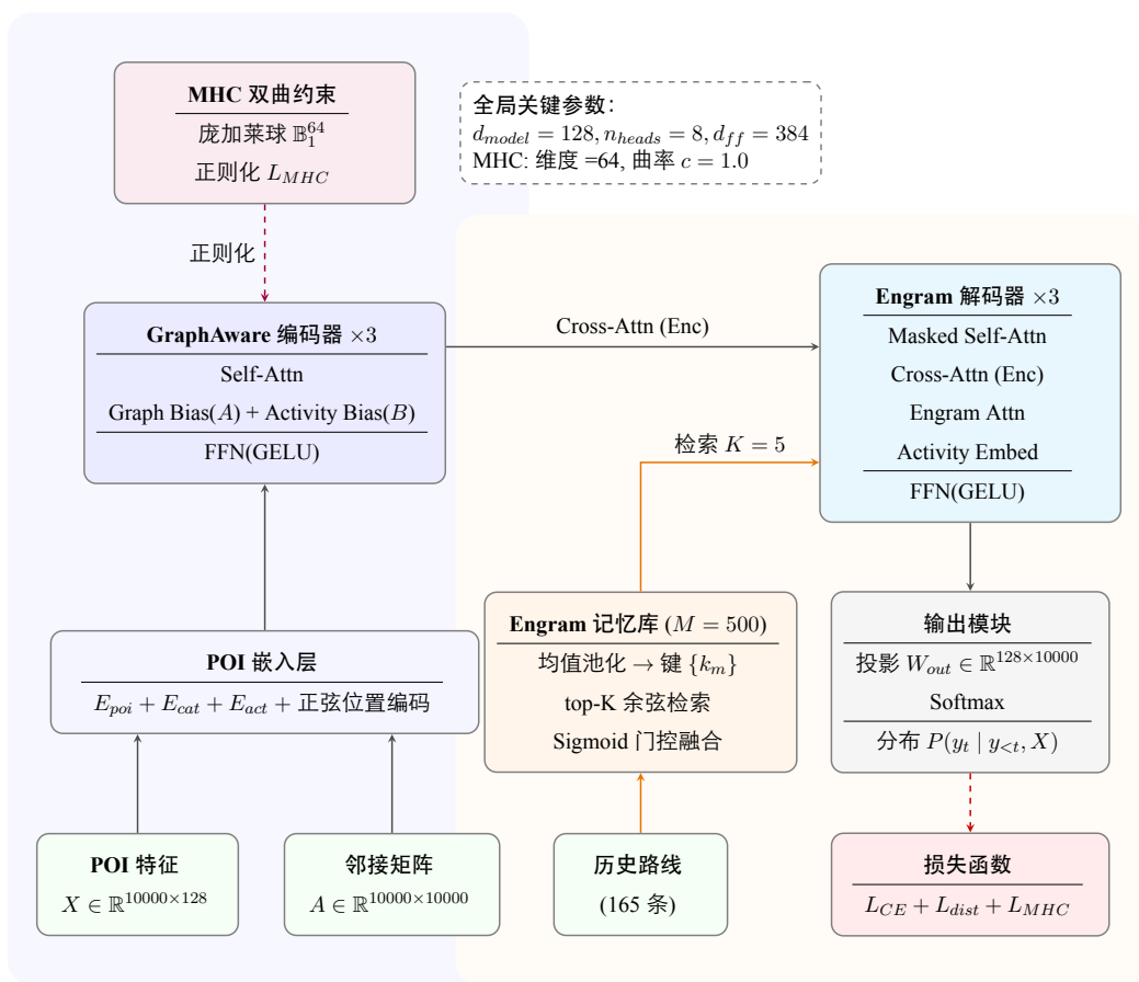
图 1 RouteTransformer 旅游路线生成模型架构图
