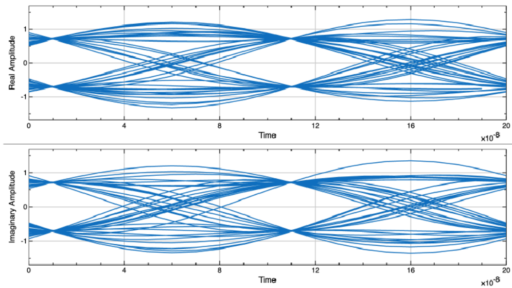
图 4 B 点眼图
