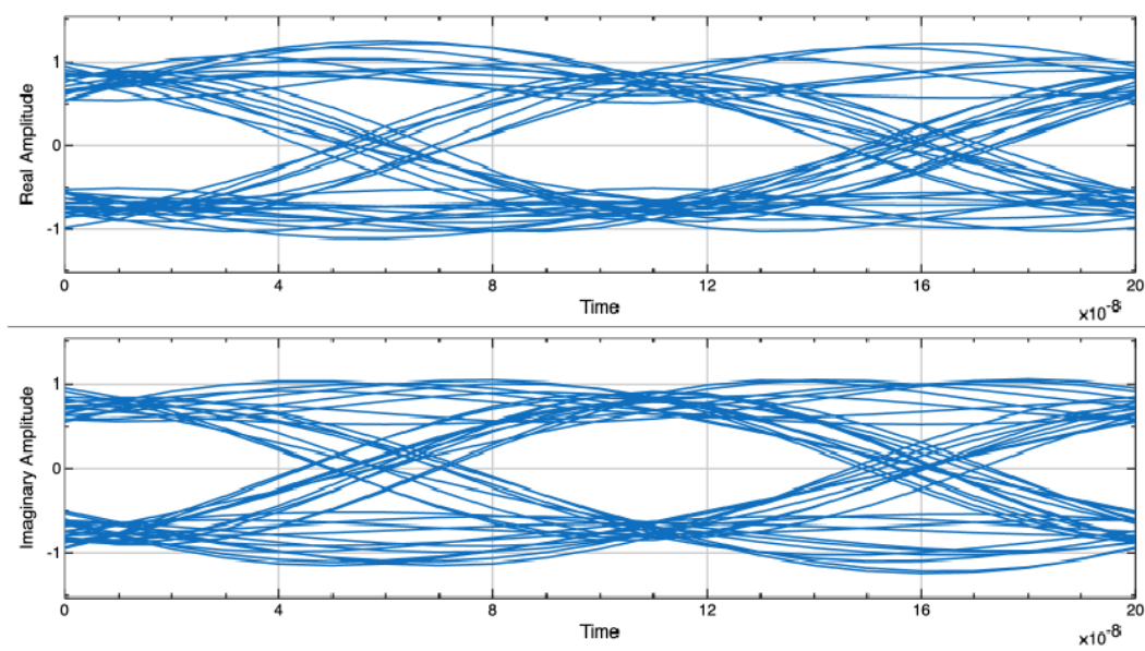
图 8 B 点眼图
