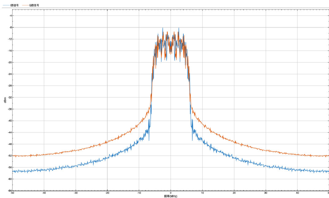
图 3 A 点频谱
