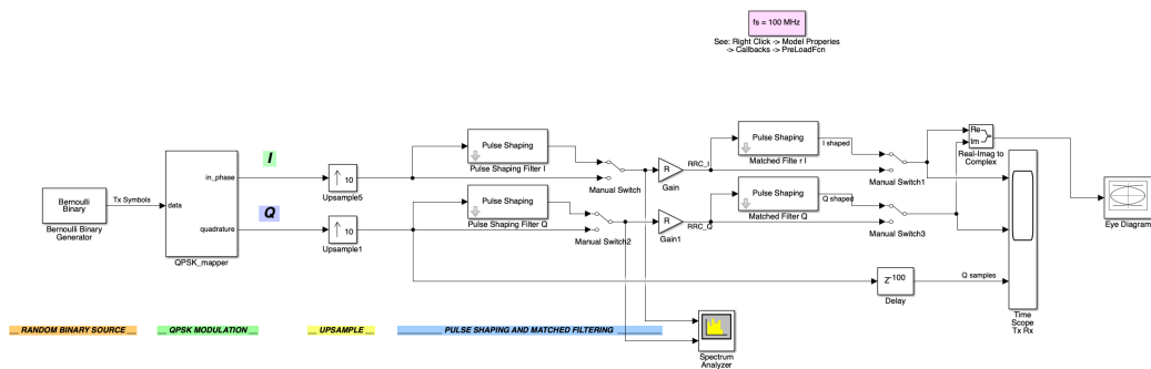
图 2 修改后的模型
