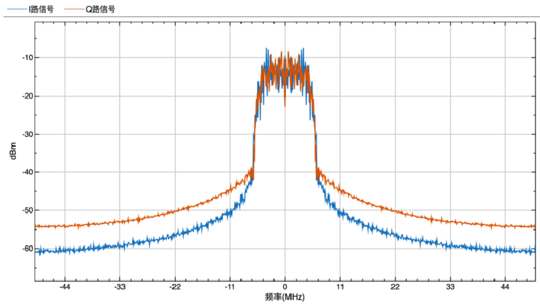
图 7 A 点频谱
