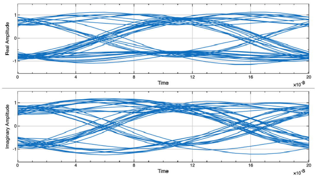
图 6 B 点眼图
