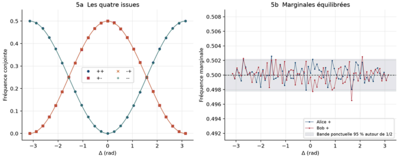
Figure 5. Les quatre fréquences conjointes suivent la loi normalisée tandis que les deux marginales fluctuent autour de 1/2 . Les courbes ++ et -- , ainsi que +- et -+ , se superposent théoriquement. La bande grise est ponctuelle ; ce n'est pas une bande simultanée couvrant toute la grille.
